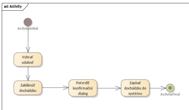
Figure 2: Diagram aktivít zapisovania dochádzky
