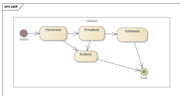
Figure 1: Stavový diagram vytvárania udalosti
