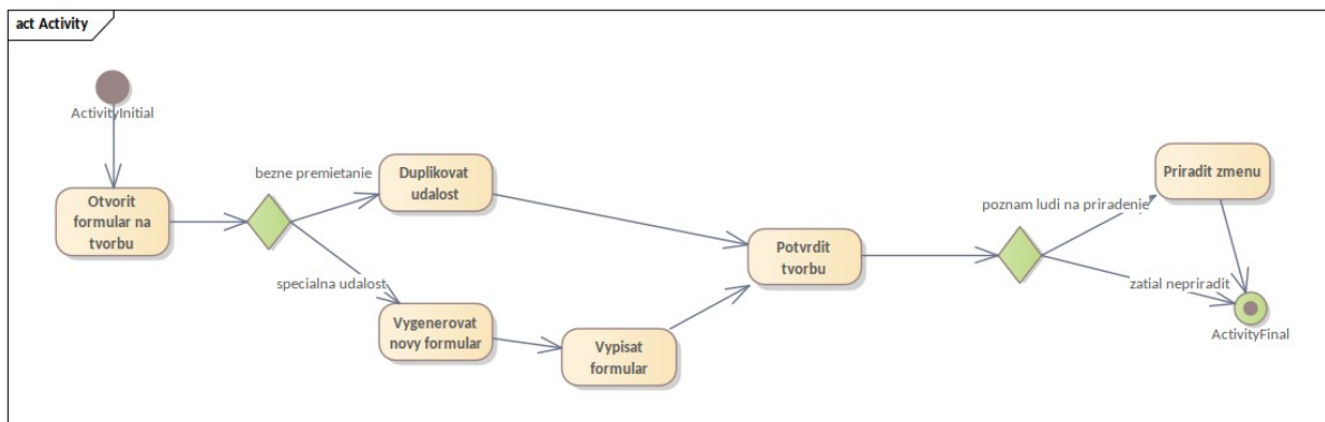
Figure 3: Diagram aktivít tvorby udalosti
