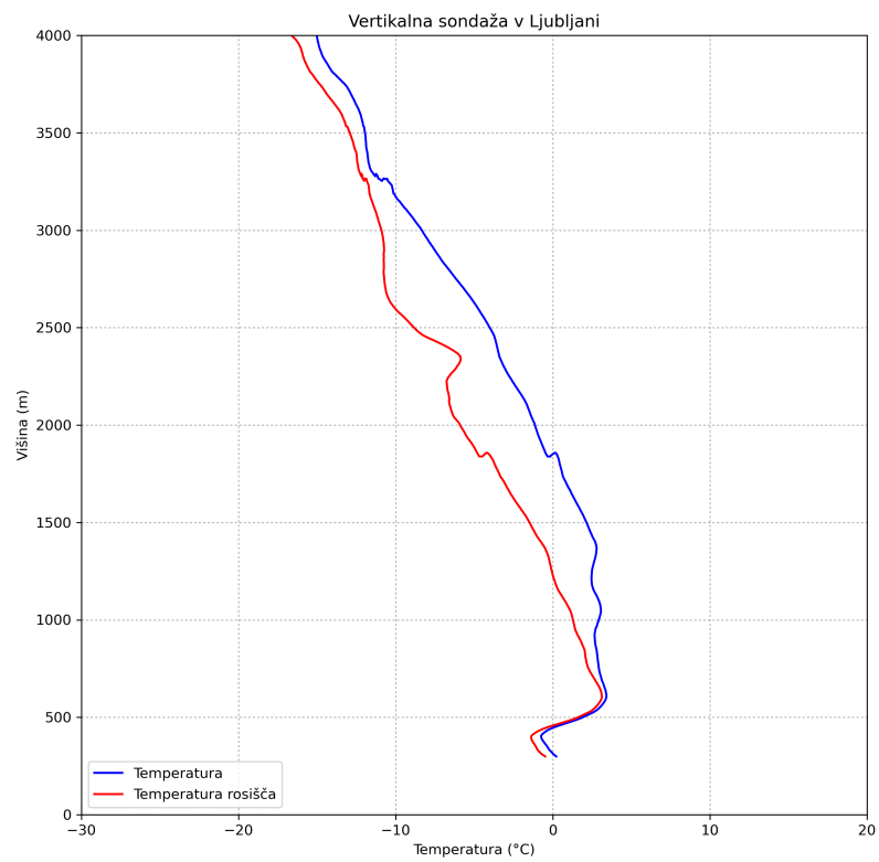
Figure 1: Radiosondaža izrisana s pomočjo pythonom
