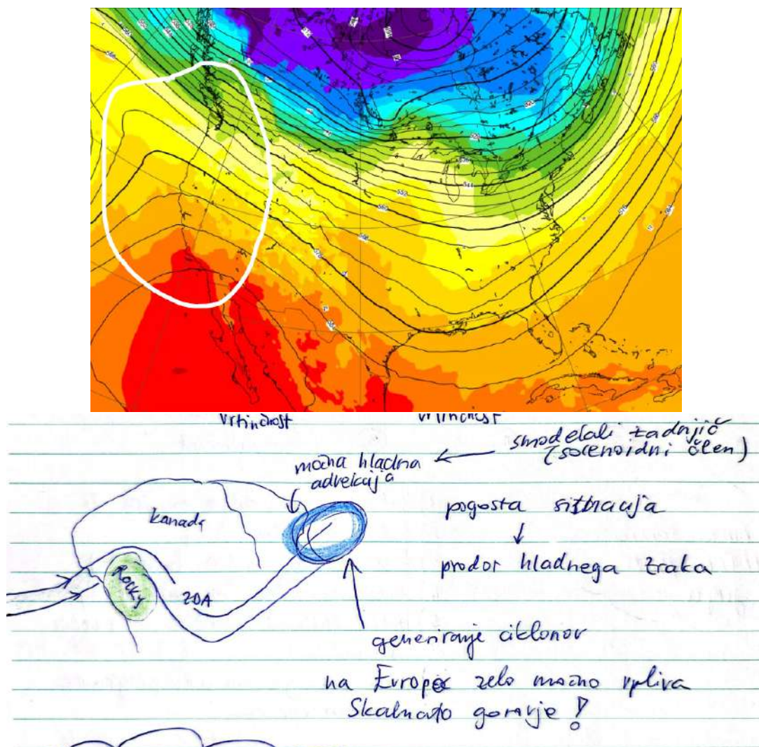
Slika 17.27: Valovi v območju Skalnega gorovja.
