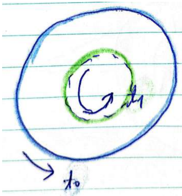
Slika 17.16: Zmanjšanje radija.
