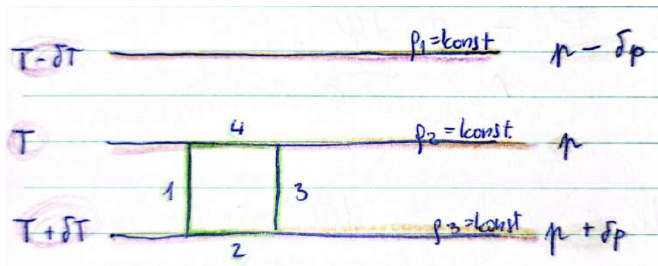
Slika 17.5: Integracijska zanka v barotropni atmosferi.
