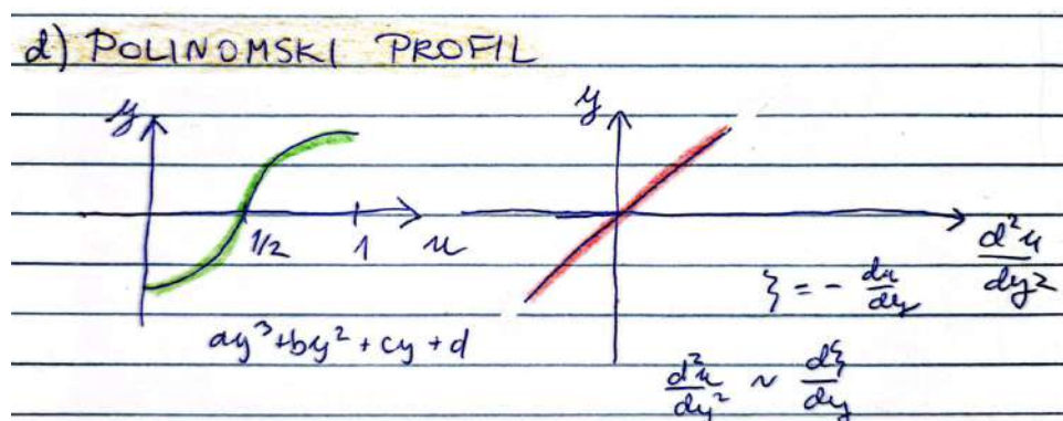
Slika 19.10: Primer polinomskega profila osnovnega toka (levo) in skica drugega odvoda oziroma gradienta osnovne vrtinčnosti za polinomski profil (desno).
