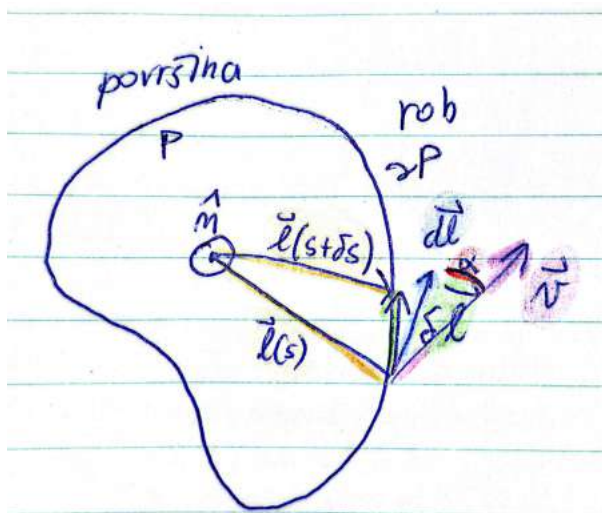
Slika 17.10: Skica za izračun cirkulacije Zemlje.
