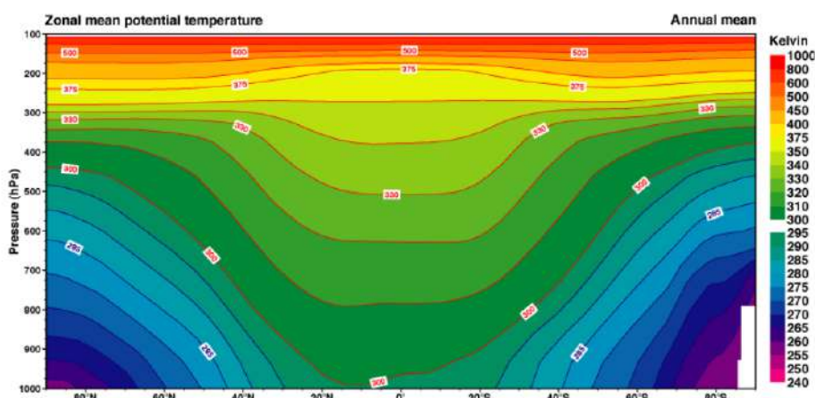
Slika 7.18: Potencialna temperatura, povprečena po zonali.
