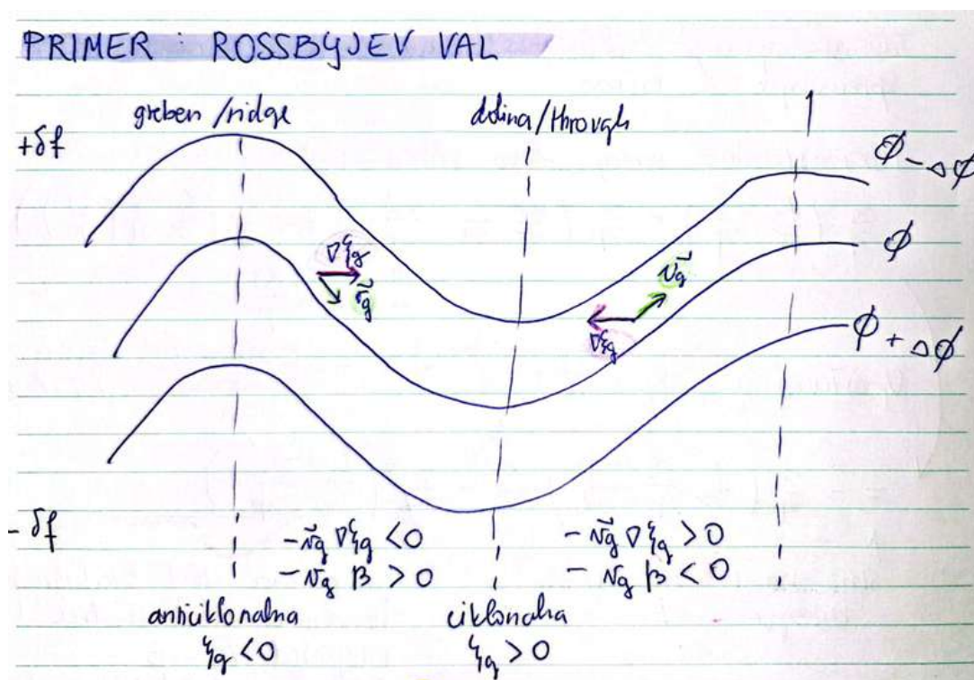
Slika 18.12: Skica Rossbyjevega vala z grebenom, dolino, geostrofskim vetrom in gradientom geostrofske vrtinčnosti.
