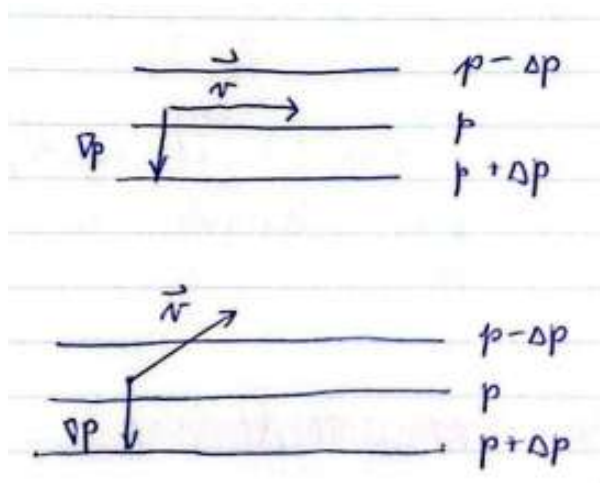
Slika 7.13: Če je veter vzporeden z izobarami, je \vec{v} \cdot \nabla p = 0 in sila gradienta tlaka ne opravlja dela.
