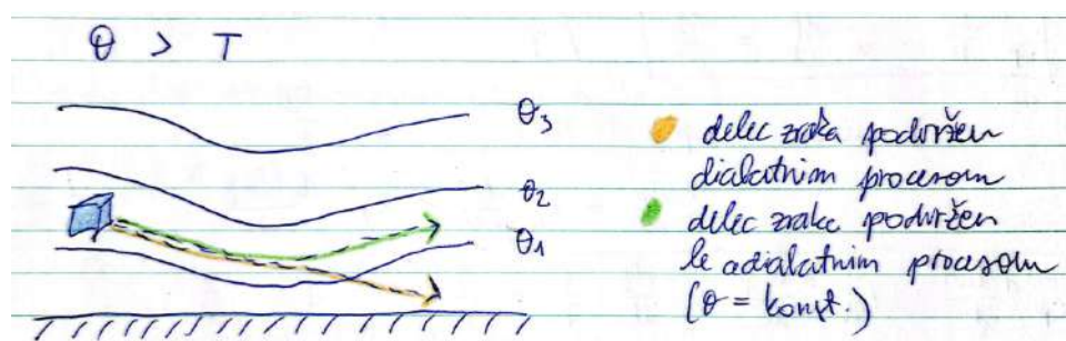
Slika 7.16: Gibanje delca po izentropah in med njimi.
