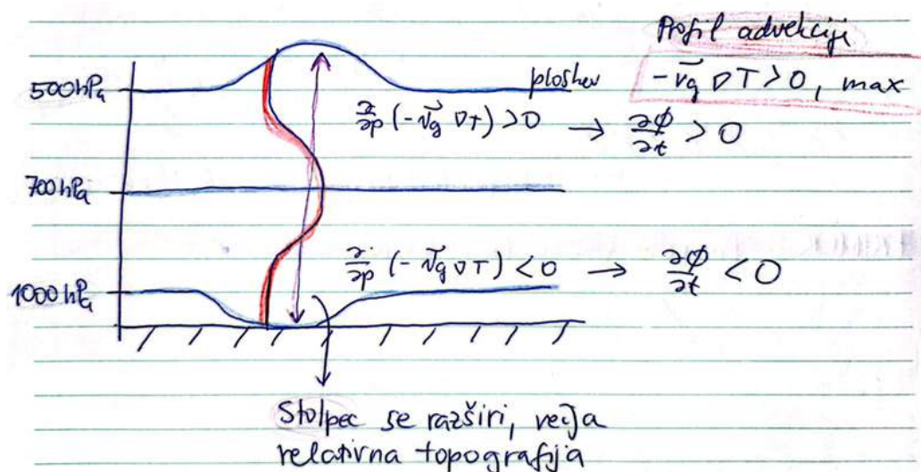
Slika 18.13: Skica vertikalnega profila tople advekcije z maksimumom v spodnji oziroma srednji troposferi.
