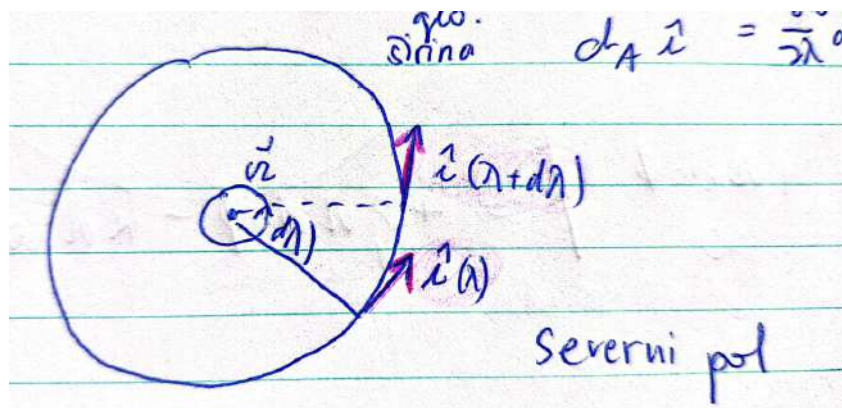
Slika 7.2: Spreminjanje lokalnega baznega vektorja \vec{i} zaradi vrtenja Zemlje.
