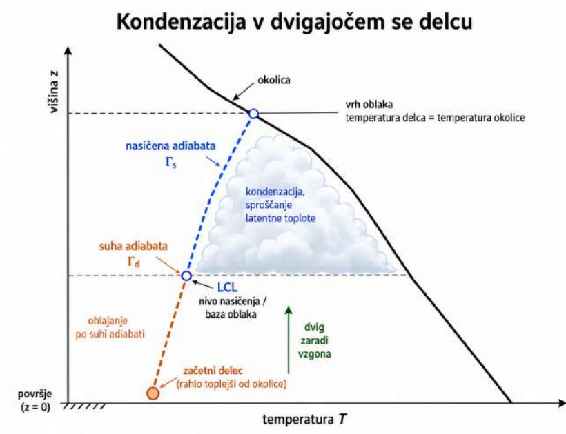
Slika 11.7: Dvignjeni delec, LCL in nadaljnje gibanje po nasičeni adiabat.
