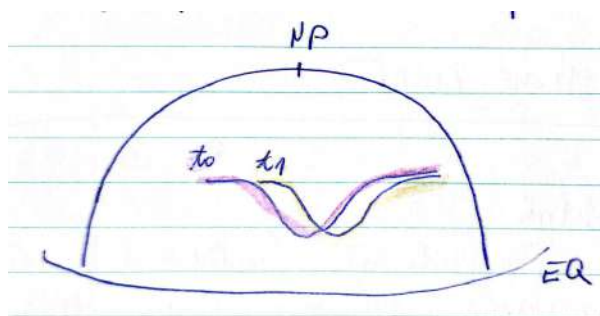
Slika 17.40: Skica kratkih valov.
