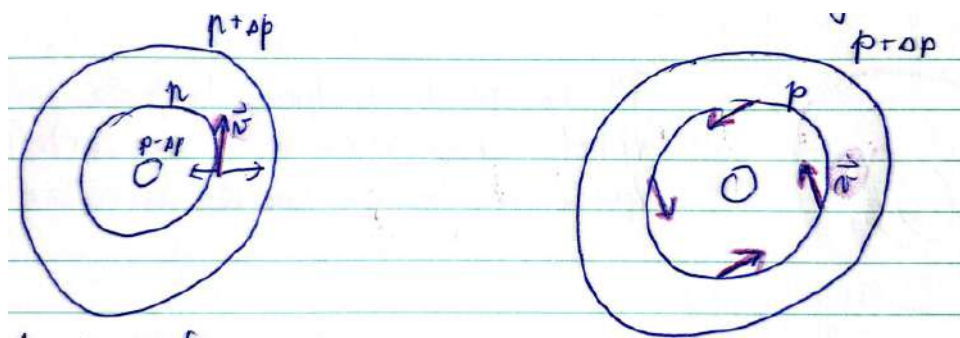
Slika 17.18: Srednja troposfera (desno) in spodnja troposfera (levo).
