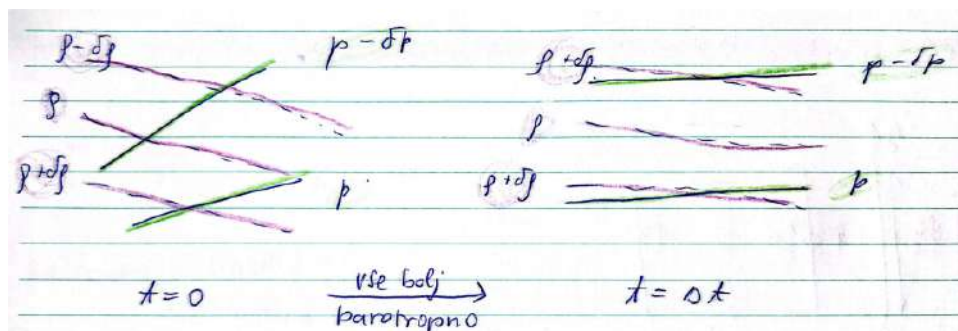
Slika 17.12: Izolinije gostote se bodo premaknile tako, da bodo bolj vzporedne z izobarame.
