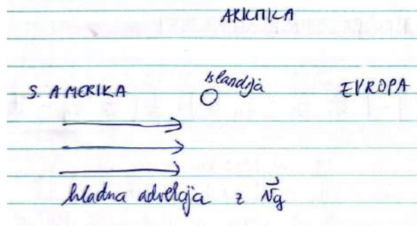
Slika 17.22: Skica območja ciklogeneze
