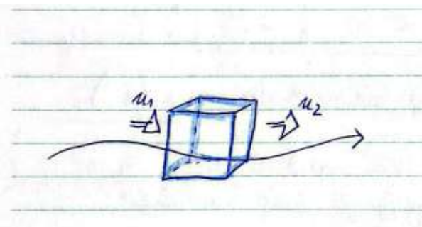
Slika 7.10: Skica k Lagrangeovski izpeljavi kontinuitetne enačbe.
