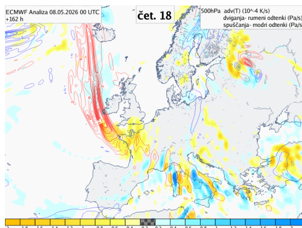
Slika 18.24: Primer lokalnega maksimuma tople advekcije južno od Irske. S tem je povezano območje dviganja, prikazano z rumenimi odtenki.
