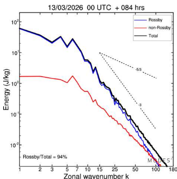
Slika 17.34: Prikaz vrha med k = 3 in k = 7 .
