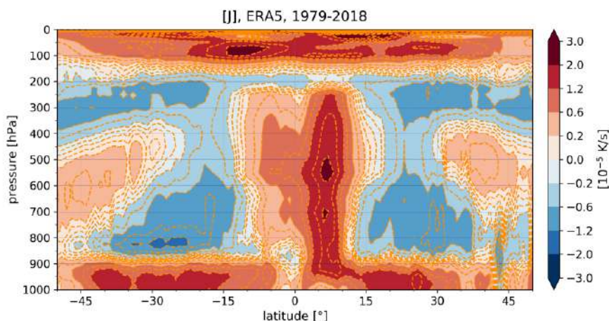
Slika 7.20: Povprečno diabatno gretje v reanalizi ERA5 za obdobje 1979–2018.
