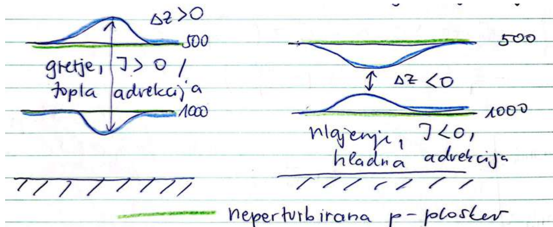
Slika 18.14: Vpliv diabatskega gretja in hlajenja na debelino plasti med izobarnima ploskvama. Levo gretje, desno hlajenje.
