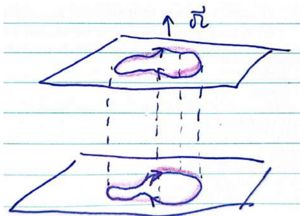
Slika 16.2: Barotropna atmosfera.
