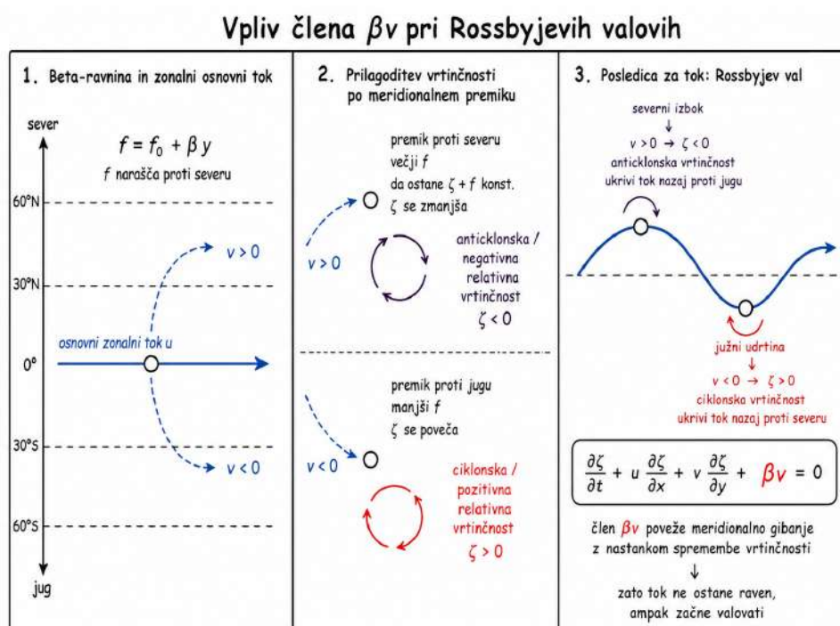
Slika 17.31: Rossbyev val.
