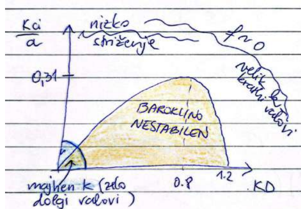
Slika 19.16: Skica rasti Eadyjeve barokline motnje. Rast je največja pri približno KD \approx 0.8 , nestabilnost pa izgine pri približno KD \approx 1.2 .
