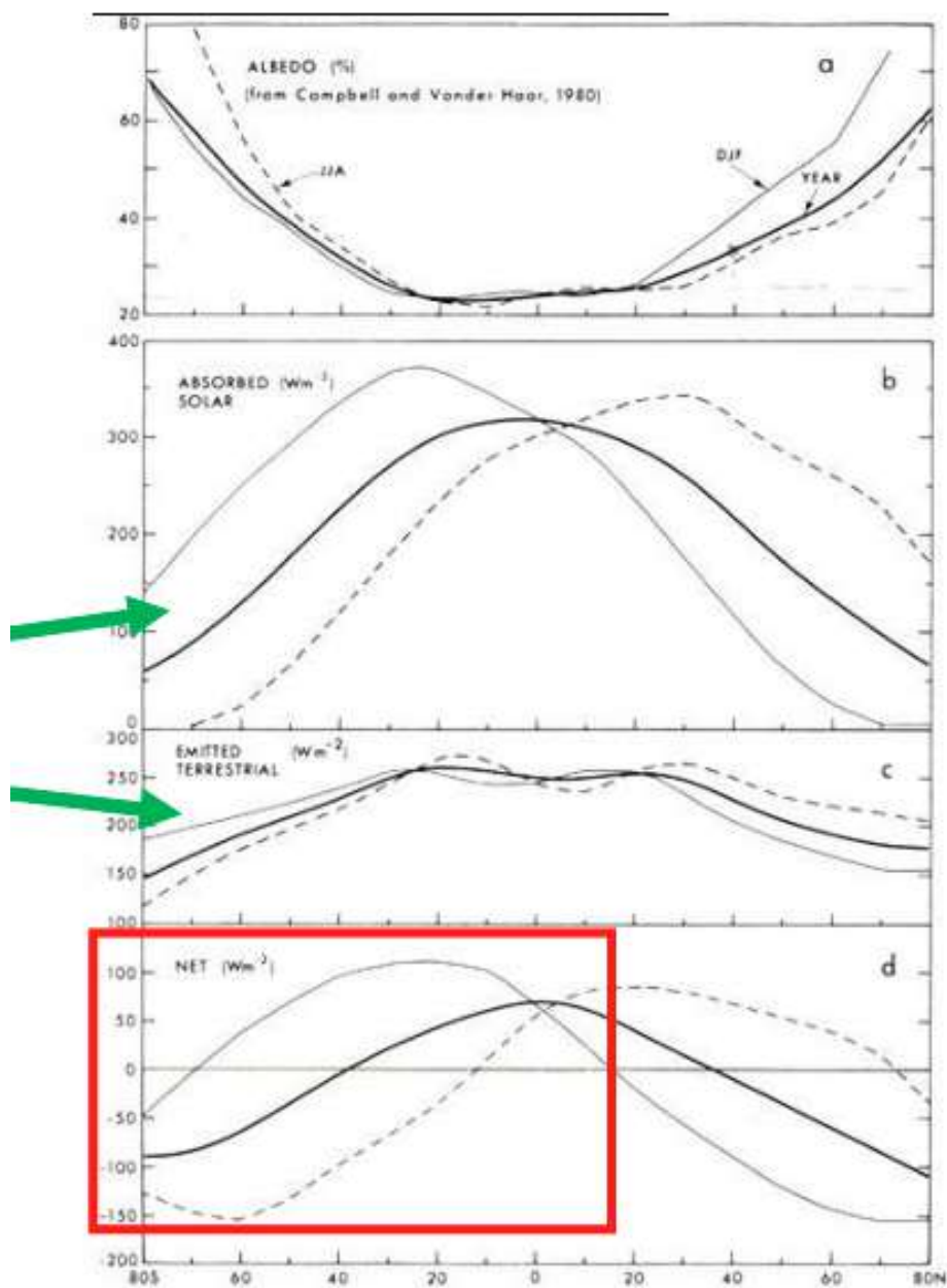
Slika 20.1: Skica energijskega neravnovesja med tropi in polarnimi predeli. Zaradi močnejšega segrevanja v tropih se vzpostavi transport toplote proti poloma.
