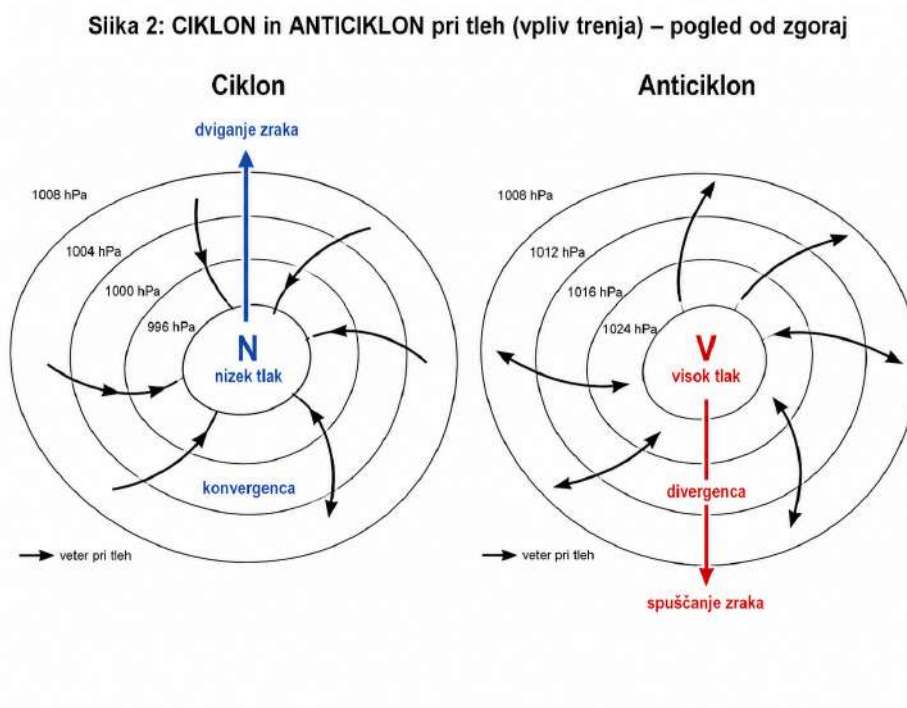
Slika 16.4: Ciklon levo, anticiklon desno.
