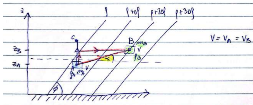
Slika 19.12: Skica nagnjenih izolinij gostote pri baroklinem stanju. Izolinije gostote niso vodoravne, zato lahko pri poševni izmenjavi dveh delcev pride do zmanjšanja potencialne energije.
