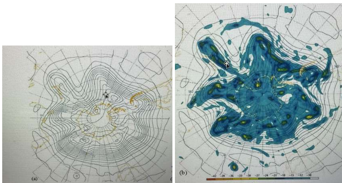
Slika 18.8: Polji geopotenciala in absolutne vrtinčnosti. Na levi strani je geopotencial, na desni strani pa absolutna vrtinčnost.
