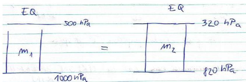
Slika 5.2: Primerjava stolpcev zraka med različnimi tlačnimi nivoji.
