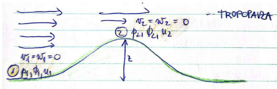
Slika 7.15: Tok čez hrib oziroma mirujoča atmosfera nad hribom.
