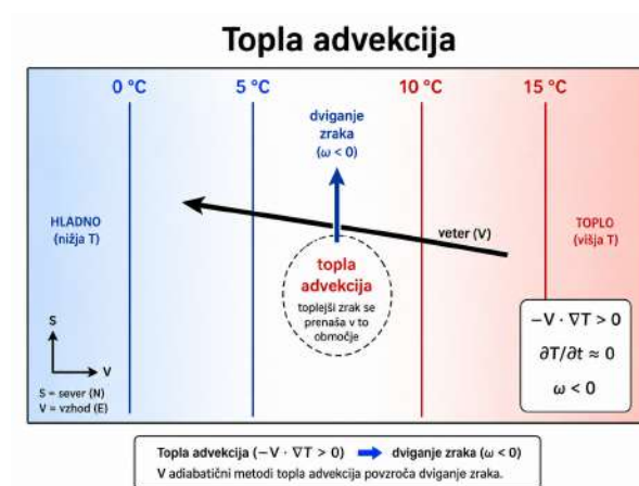
Slika 14.1: Topla advekcija.
