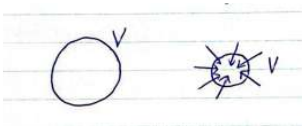
Slika 7.12: Pri divergenci se materialni volumen povečuje, pri konvergenci pa se skrči.
