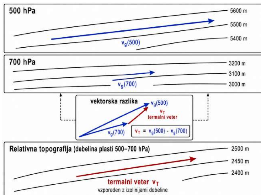
Slika 16.6: Skica geostrofskega vetra na dveh različnih višinah in pomen termalnega vetra v tem primeru.
