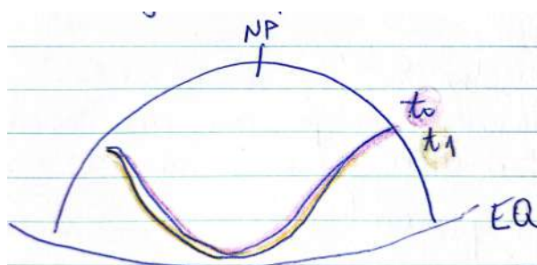
Slika 17.41: Skica dolgih valov.
