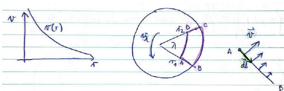
Slika 17.4: Cirkulacija v osnosimetričnem toku ( v \cdot r = \text{konst.} ).
