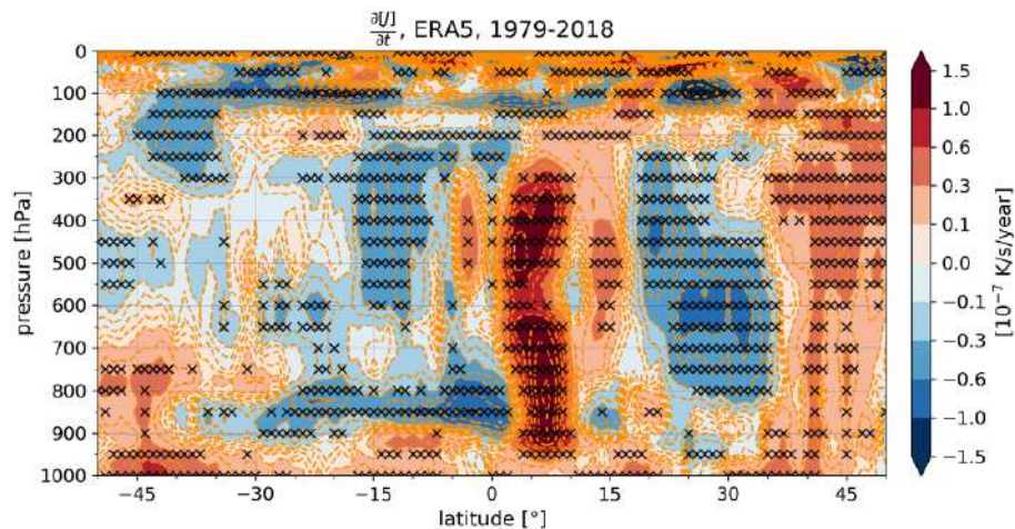
Slika 7.21: Trend diabatnega gretja v današnjem podnebjju.
