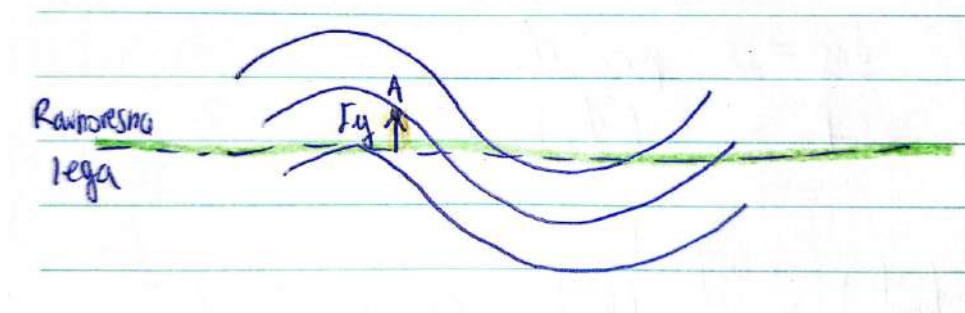
Slika 17.33: Idealiziran Rossbyjev val z oscilacijo v meridionalni smeri.
