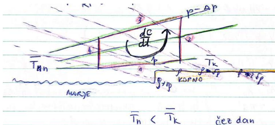
Slika 17.11: Skica cirkulacije na obali.
