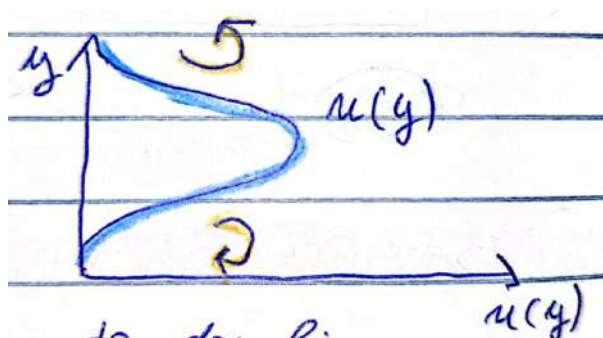
Slika 19.5: Perturbacija v osnovnem zonalnem toku U(y) , ki zaradi striženja generira anomalije vrtničnosti.
