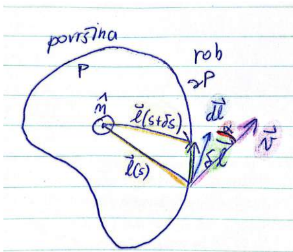
Slika 17.1: Skica fluida.
