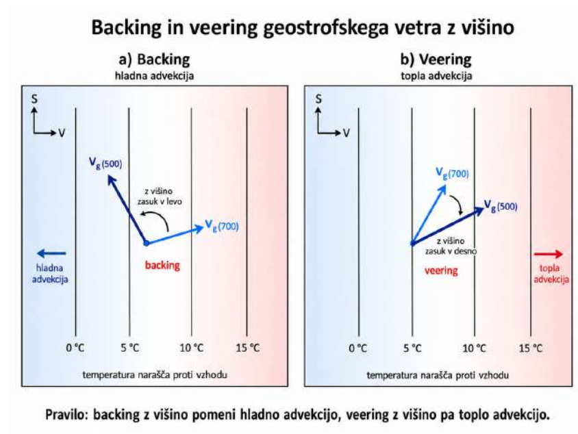
Slika 16.7: Levo backing in desno veering.
