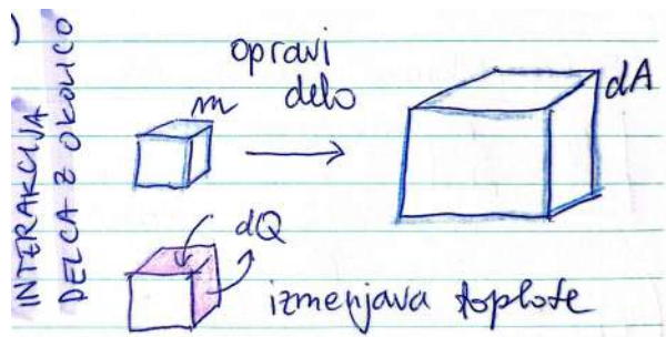
Slika 7.14: Delec zraka, ki izmenjuje toploto in opravlja delo na okolico.
