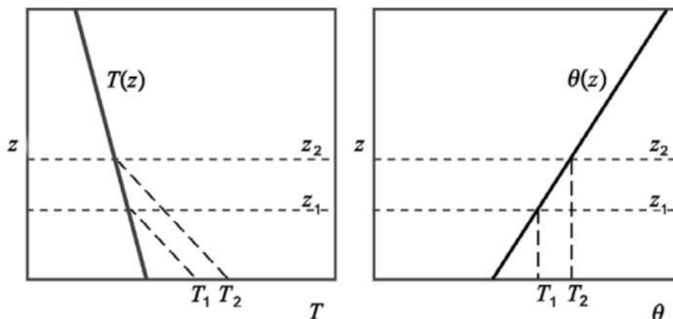
Slika 11.4: Suha konvekcija z vidika temperature (levo) in potencialne temperature (desno). Zračni delci se dvigajo s površine in sledijo suhi adiabat, dokler se njihova temperatura ne izenači s temperaturo okolja, ko postanejo nevtrarno vzgonski. Če je temperatura površine T_1 (ali T_2 ), se bo konvekcija razširila do višine z_1 (ali z_2 ). Isti postopek, gledano z vidika potencialne temperature, je enostavnejši. Stabilna plast zgoraj ima d\theta/dz > 0 ; konvekcija vrne prevrnjeno plast v stanje enakomerne \theta , ki ustreza nevtralni stabilnosti. Upoštevajte, da je po definiciji \theta = T pri p = 1000 hPa.
