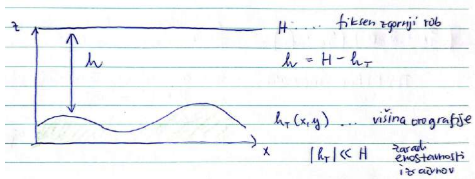
Slika 17.42: Plitva voda nad topografijo.
