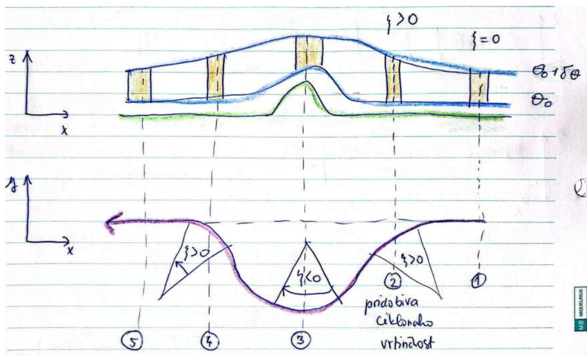
Slika 17.28: Vzhodni tok preko orografske ovire.
