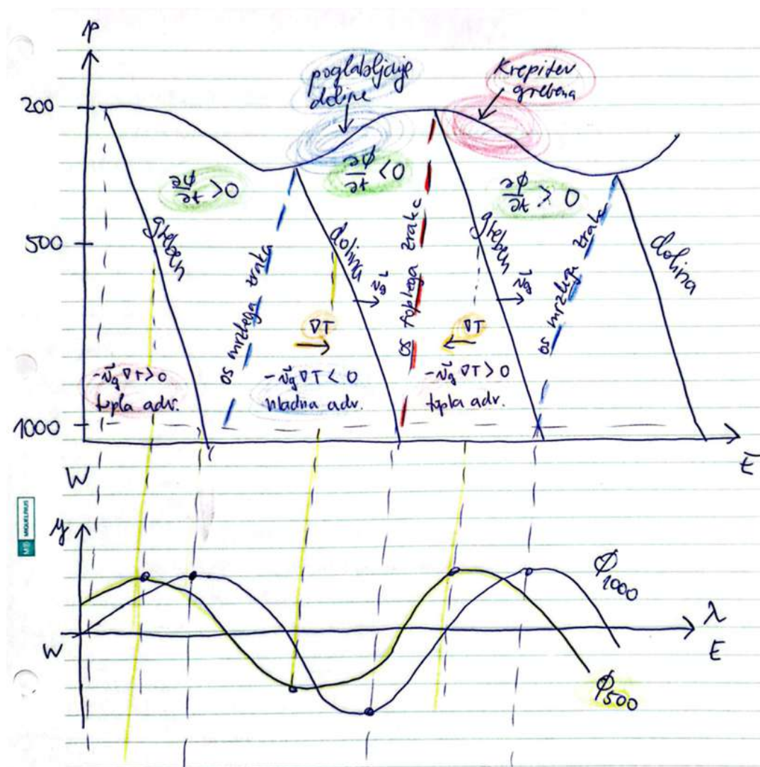
Slika 18.15: Vertikalni presek skozi baroklini val. Prikazan je nagib osi doline, osi grebena ter osi hladnega in toplega zraka.
