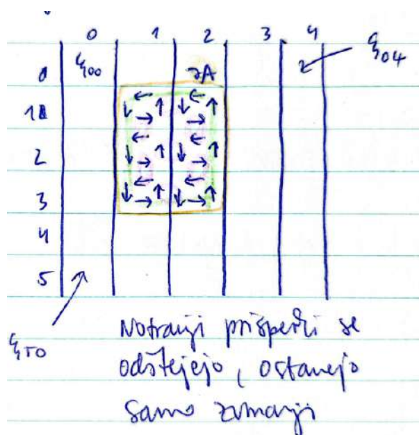
Slika 17.8: Grafični prikaz Stokesovega teorema
