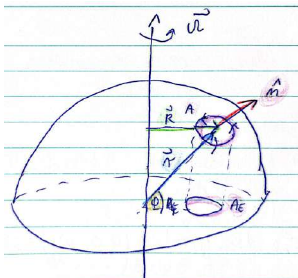
Slika 17.9: Projekcija cirkulacije na ekatorialno ravnino.
