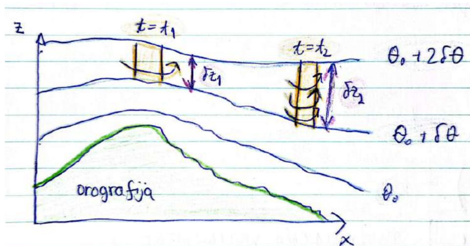
Slika 17.25: Skice za opis potencialne vrtinčnosti pri prehodu čez orografsko oviro.
