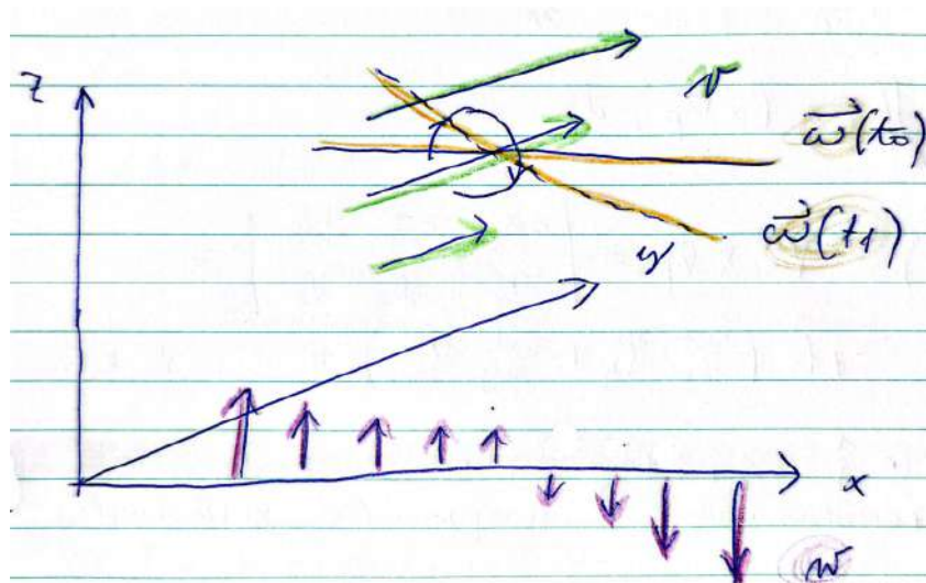
Slika 17.19: Skice za opis člena nagibanja oz. zvijanja.
