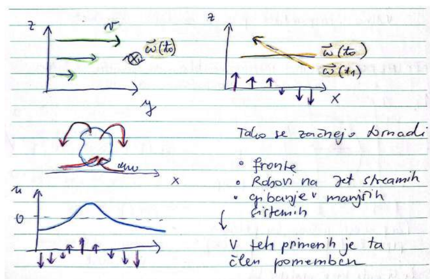
Slika 17.20: Skice za opis člena nagibanja oz. zvijanja.
