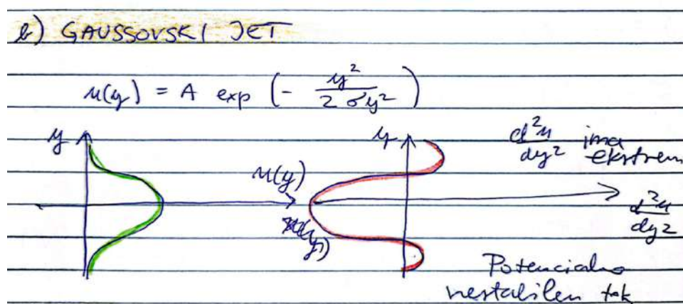
Slika 19.8: Gaussovski profil vetrovnega stržena (levo) in njegov Skicatski drugi odvod (desno).
