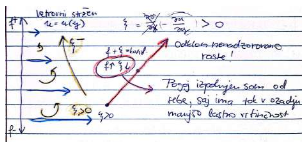
Slika 19.4: Primer zonalnega toka z močnim meridionalnim striženjem, U = U(y) .
