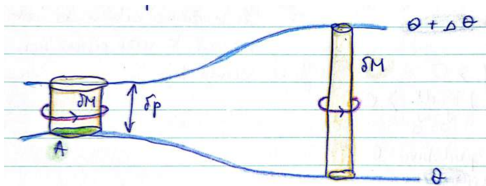
Slika 17.23: Razteg zračnega stolpca.
