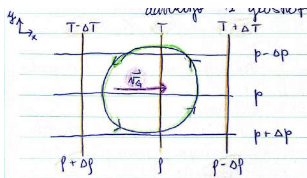
Slika 17.21: Primer: tlak in gostota sta razporejena tako, da opisujeta hladno advekcijo z geostrofskim vetrom.
