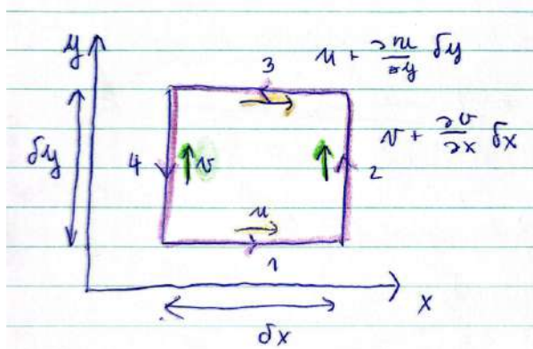
Slika 17.13: Pravokoten element fluida.
