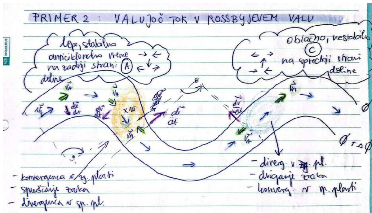
Slika 18.3: Valujoč tok v Rossbyjevem valu.
