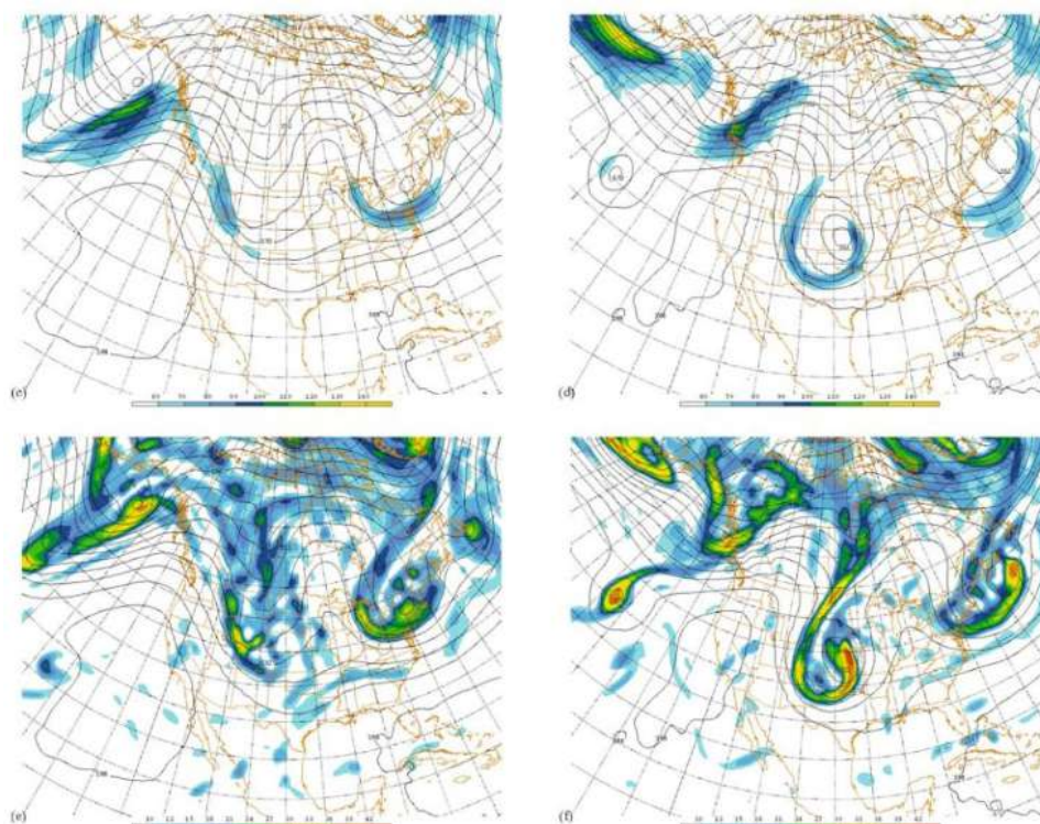
Slika 18.20: Primer močnejšega toka na zahodni oziroma gorvodni strani doline. S tem je skladno tudi polje vrtničnosti. Člen B v tem primeru deluje tako, da advektira pozitivno vrtničnost, zato je B > 0 . Vrtničnost v dolini se poveča, dobimo \frac{\partial \Phi}{\partial t} < 0 , dolina se poglobi, hkrati pa se translira proti ekvatorju.
