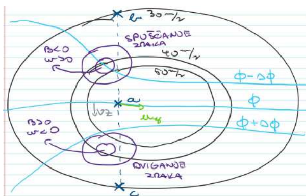
Slika 18.26: Presek skozi jet stream med hladnejšim in toplejšim stolpcem ter pripadajoča ageostrofska cirkulacija.
