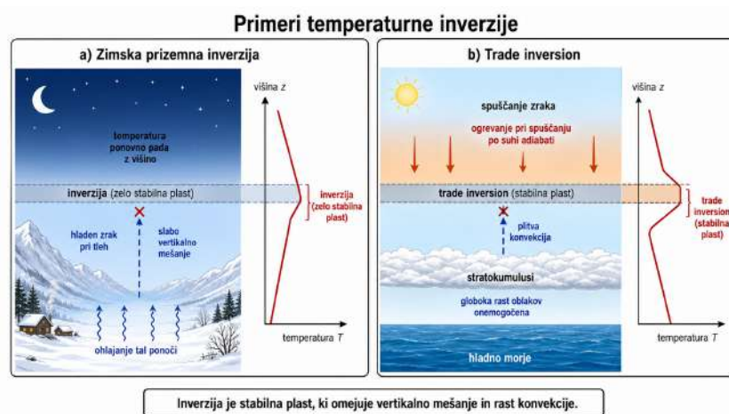
Slika 11.6: Primeri inverzije: zimska prizemna inverzija in trade inversion.
