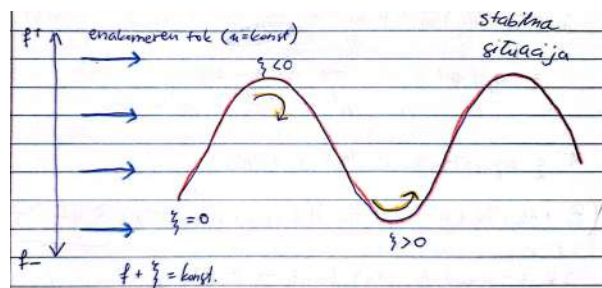
Slika 19.3: Stabilen primer Rossbyjevega vala v enakomernem zonalnem toku, kjer je osnovni povratni mehanizem \beta -efekt.
