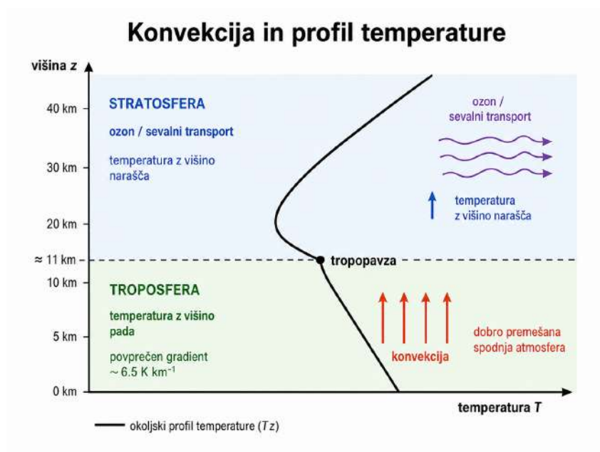
Slika 11.3: Konvekcija in profil temperature.
