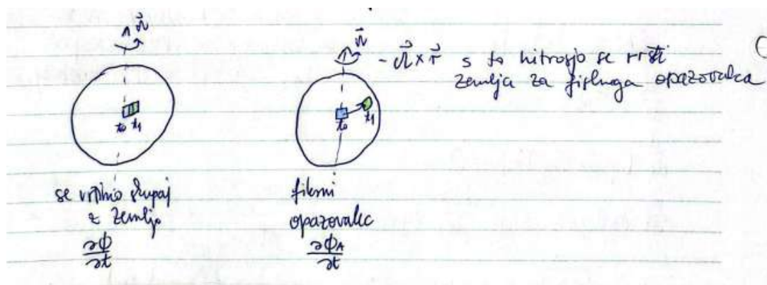
Slika 7.11: Opazovanje skalarne polja v absolutnem in relativnem sistemu.
