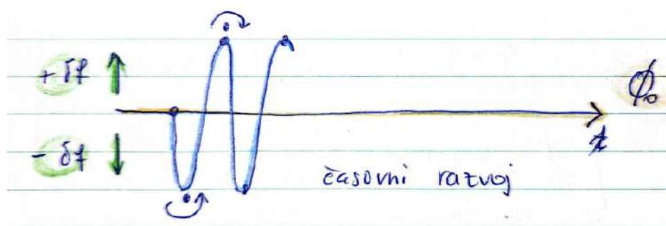
Slika 18.10: Mehanizem Rossbyjevega vala: odklon delca in izmenjava med planetarno ter relativno vrtničnostjo.
