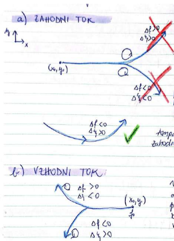
Slika 17.30: Zahodni tok (zgoraj) in vzhodni tok (spodaj).
