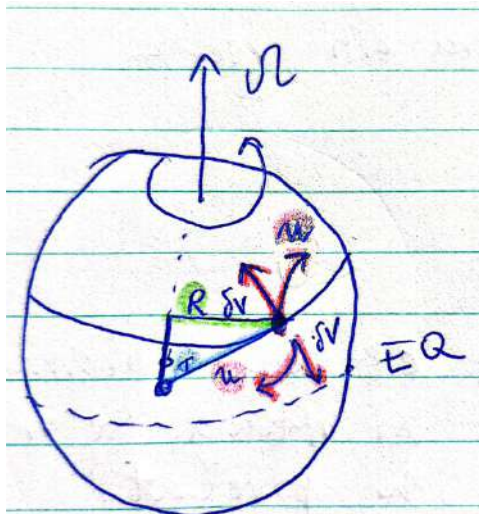
Slika 6.11: Gibanje delca proti severu in ohranitev vrtilne količine.
