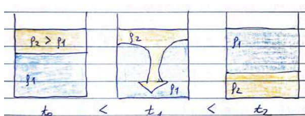
Slika 19.1: Skica statično nestabilne razporeditve, kjer je gostejša tekočina nad redkejšo.
