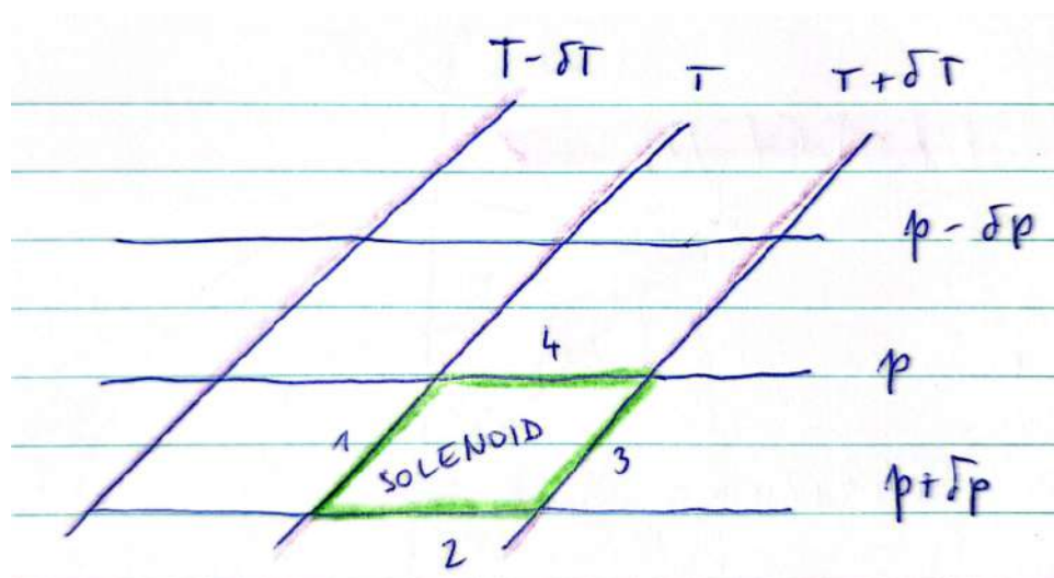
Slika 17.6: Integracijska zanka v baroklini atmosferi.
