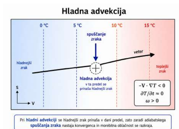
Slika 14.2: Hladna advekcija.
