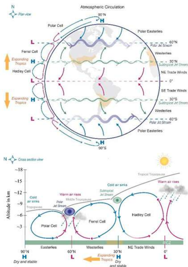
Slika 20.2: Skica treh glavnih meridionalnih cirkulacijskih celic na vsaki polobli. Hadleyjeva celica zavzema tropske predele in je omejena zaradi vpliva vrtenja Zemlje.
