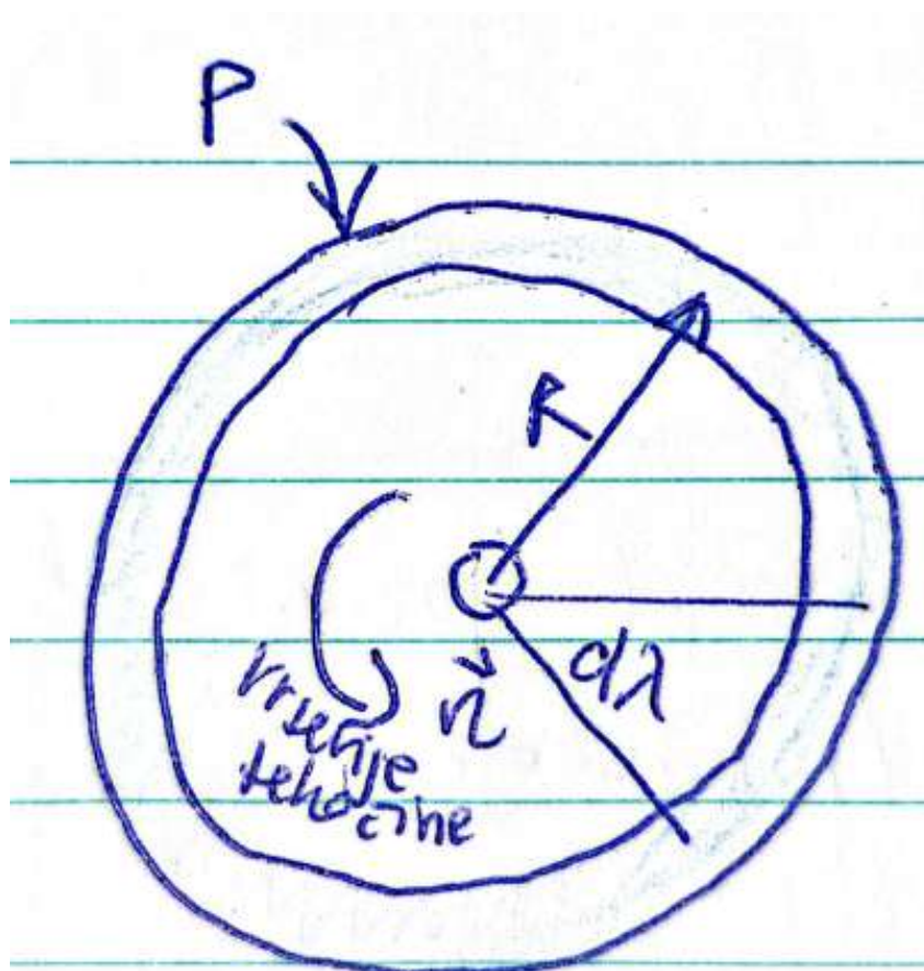
Slika 17.3: Cirkulacija v primeru rotacije tekočine po obodu z radijem R .
