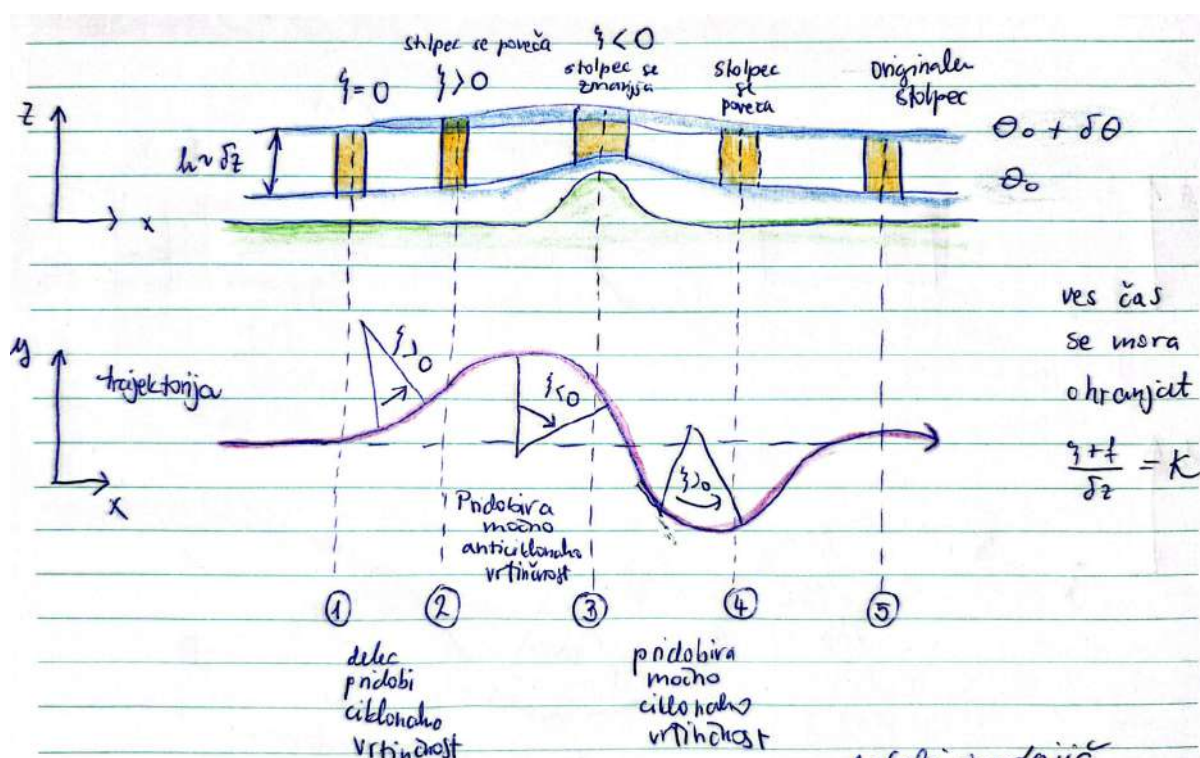
Slika 17.26: Zahodni tok preko orografske ovire.
