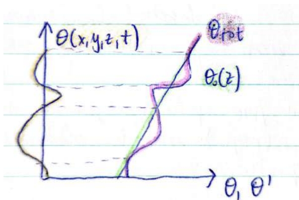
Slika 7.17: Osnovno stanje plus deviacija od tega stanja.
