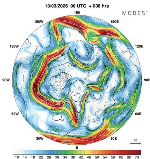
Slika 17.38: Primer zelo dolgega Rossbyjevega vala.
