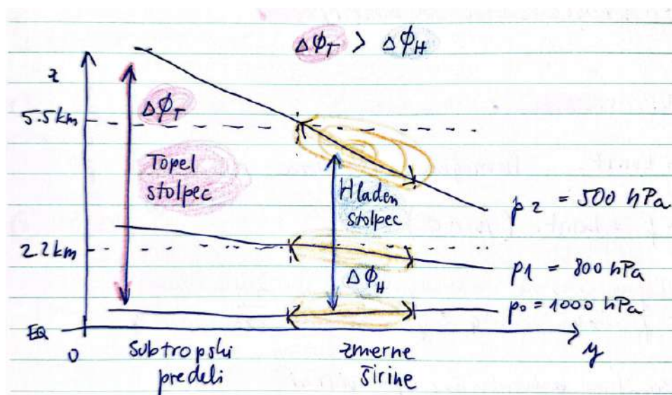
Slika 16.5: Skica geostroskega vetra na različnih višinah.
