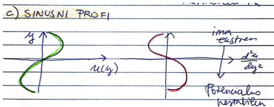
Slika 19.9: Sinusni profil osnovnega toka (levo) in njegov drugi odvod (desno).
