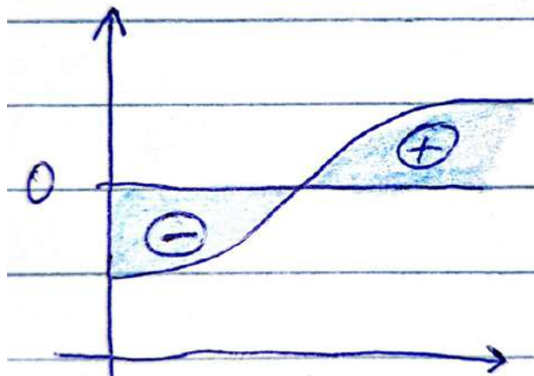
Slika 19.6: Skica funkcije, katere integral je lahko enak nič samo, če ima v domeni pozitivne in negativne prispevke.
