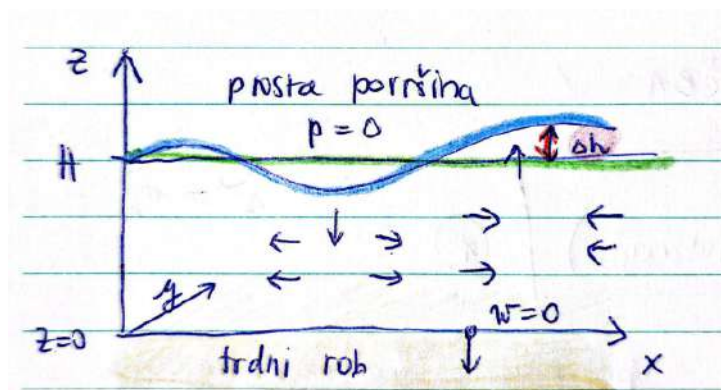
Slika 17.29: Skica za enačbe plitve vode.
