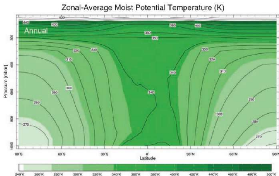
Slika 11.2: Zonalno povprečje ekvivalentne potencialne temperature.
