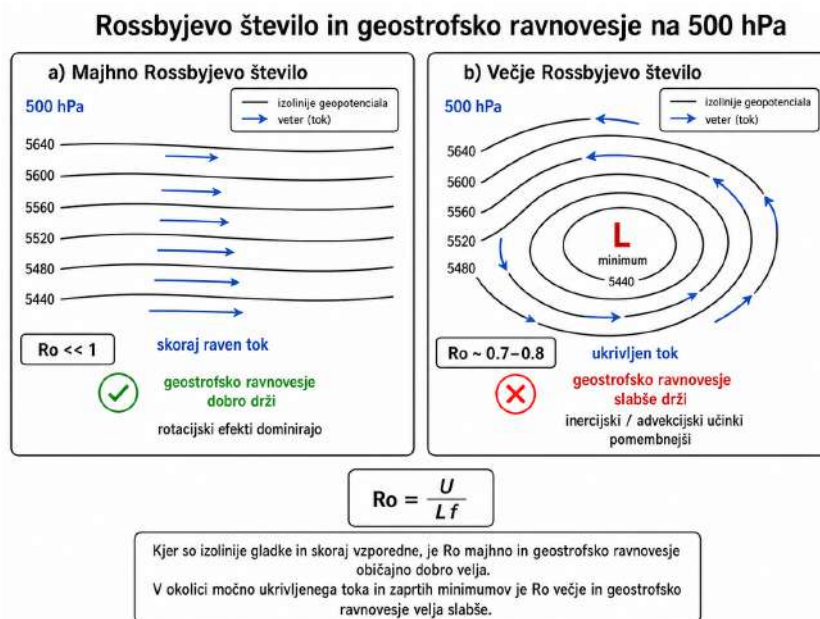
Slika 16.1: Rossbyjevo število na 500 hPa ploskvi.
