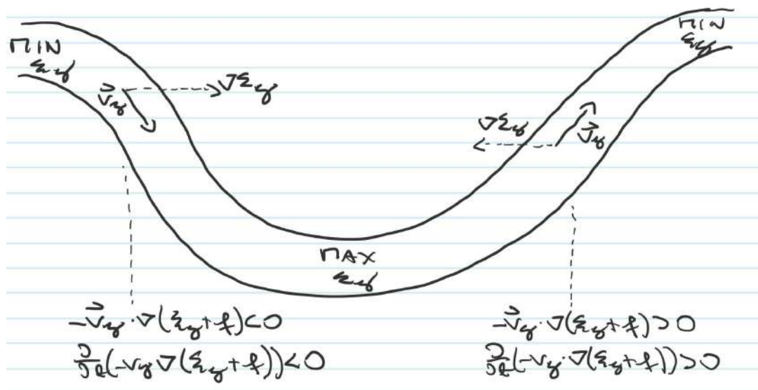
Slika 18.23: Skica Rossbyjevega vala z dolino, grebenom, geostrofskim vetrom in poljem relativne vrtinčnosti.
