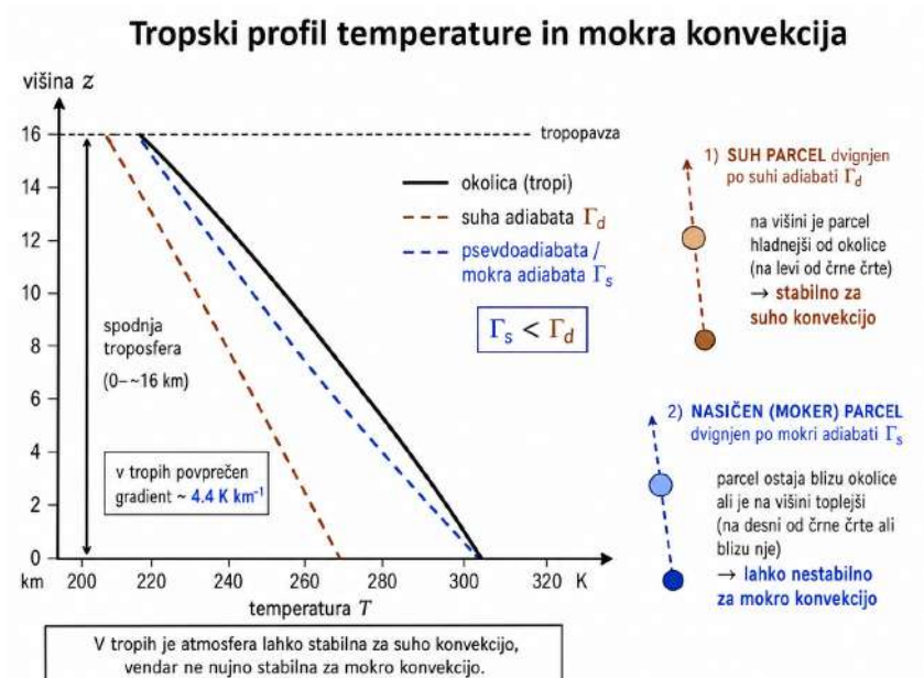
Slika 11.5: Tropski profil temperature in mokra konvekcija.
