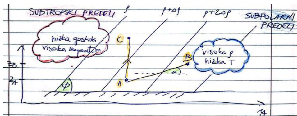
Slika 19.11: Skica baroklinega osnovnega stanja z nagnjenimi izolinijami gostote oziroma potencialne temperature.
