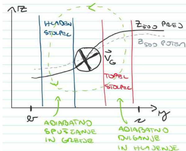
Slika 18.27: Razporeditev spuščanja in dviganja zraka ob jet streamu, ki pomaga obnoviti ravnovesje termalnega vetra.
