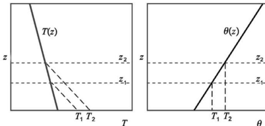
Slika 7.19: Suha konvekcija, gledana z vidika temperature in potencialne temperature.
