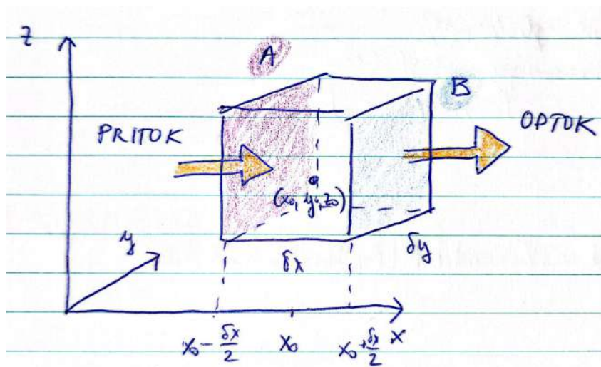
Slika 7.9: Kontrolni volumen za izpeljavo zakona o ohranitvi mase.
