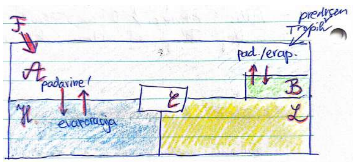
Slika 2.1: Podnebni sistem.
