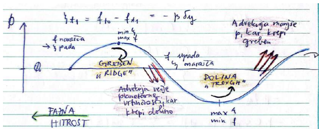
Slika 17.32: Skica ohranitve absolutne vrtnčnosti pri meridionalnem odmiku delca.
