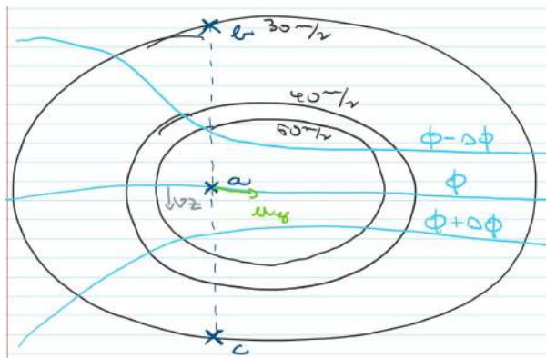
Slika 18.25: Skica konfluentnega zahodnega jet streama z izohipsami in izotahami.
