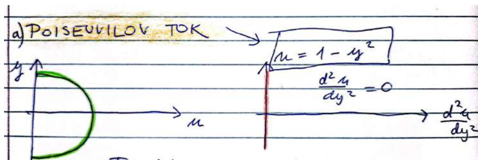
Slika 19.7: Poiseuilleov profil osnovnega toka U(y) = 1 - y^2 (levo) in njegov drugi odvod (desno).
