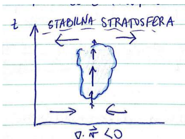
Slika 17.15: Nastanek tropskega ciklona
