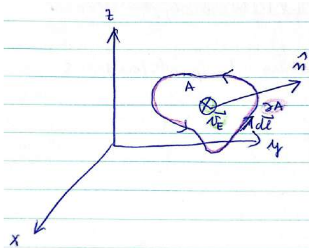
Slika 17.7: Skica za Stokesov teorem
