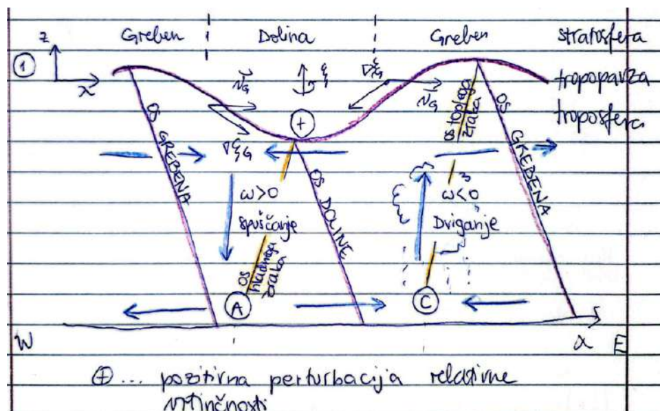
Slika 19.13: Skicatski vertikalni presek Rossbyjevega vala. Os z kaže navzgor, os \lambda pa v smeri geografske dolžine. Prikazana sta nagnjena os doline in grebena ter lega tropopavze.
