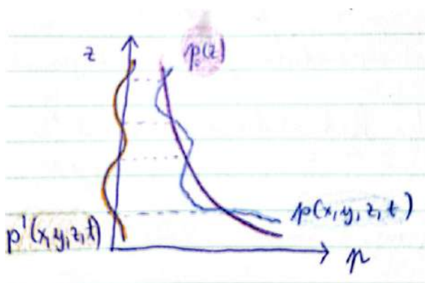
Slika 7.8: Razcep tlačnega polja na povprečen profil in perturbacijo.
