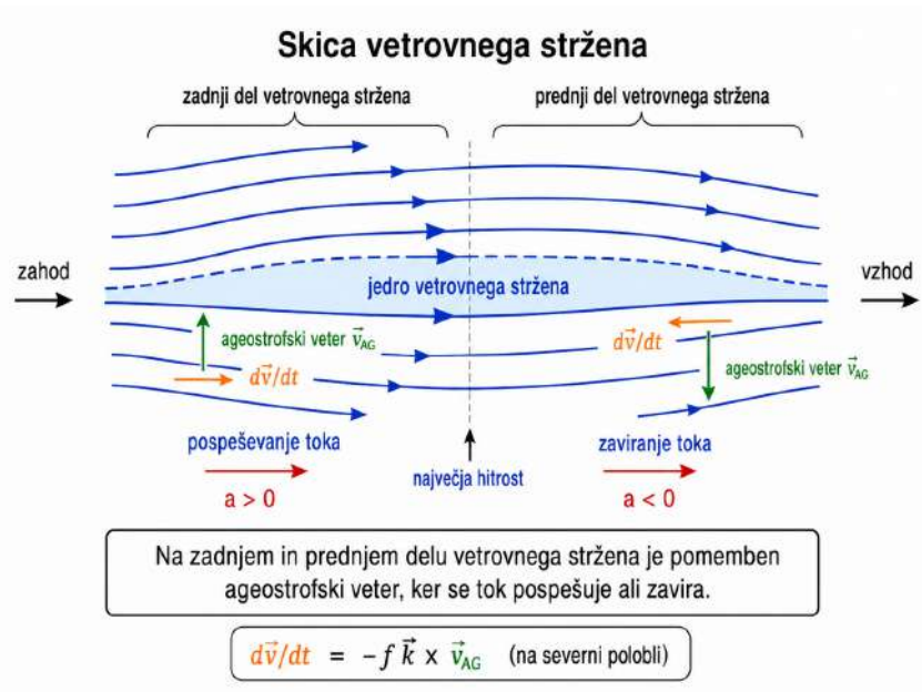
Slika 7.7: Skica vetrovnega stržena.
