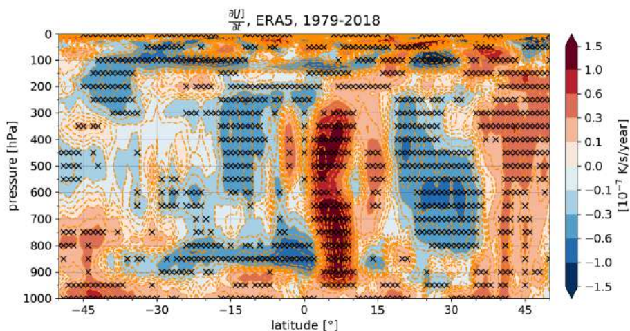
Slika 7.21: Trend diabatnega gretja v današnjem podnebnju.
