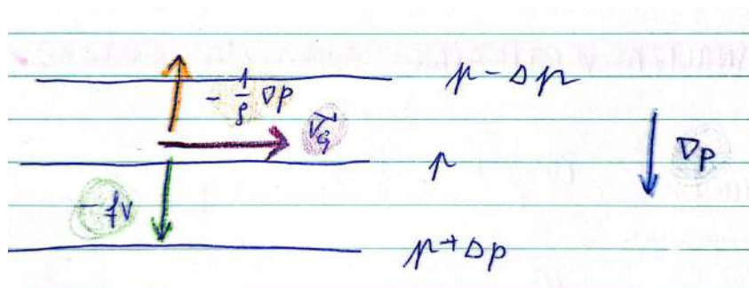
Slika 7.6: Skica izobar in geostrofskega vetra.
