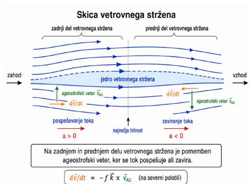
Slika 7.7: Skica vetrovnega stržena.
