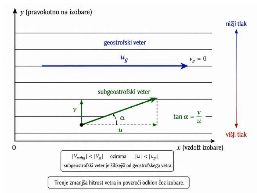
Slika 15.4: Skica k izpeljavi.
