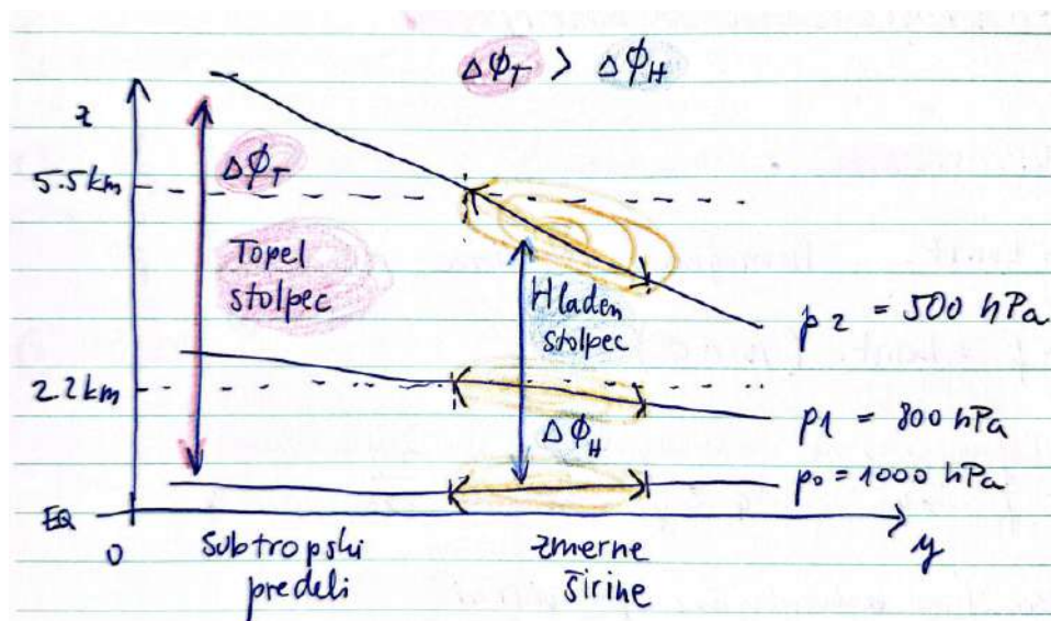
Slika 15.6: Skica geostrofskega vetra na različnih višinah.
