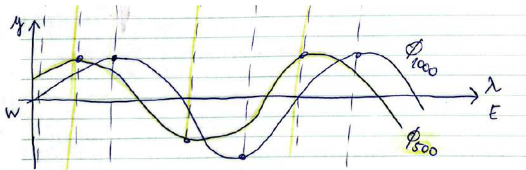
Slika 17.16: Horizontalni prikaz baroklinega vala na različnih tlačnih ploskvah. Polje geopotenciala je z višino fazno zamaknjeno.
