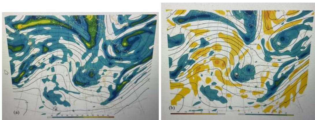
Slika 17.9: Absolutna vrtničnost na severni polobli in relativna vrtničnost v okolici Floride.
