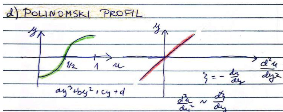
Slika 18.12: Primer polinomskega profila osnovnega toka. Na sliki je prikazan tudi njegov drugi odvod oziroma gradient osnovne vrtinčnosti.
