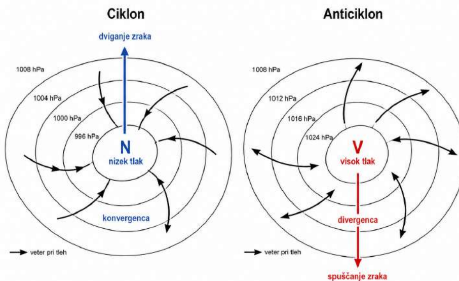
Slika 2: CIKLON in ANTICIKLON pri tleh (vpliv trenja) – pogled od zgoraj
