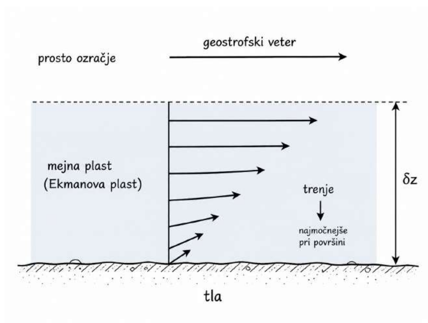
Slika 15.3: Skica mejne plasti oziroma Ekmanove plasti.
