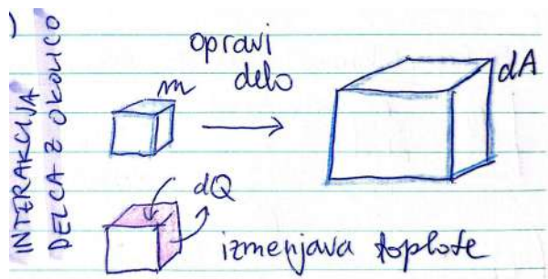
Slika 7.14: Delec zraka, ki izmenjuje toploto in opravlja delo na okolico.
