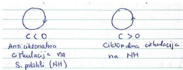
Slika 16.2: Orientacija cirkulacije na severni polobli.
