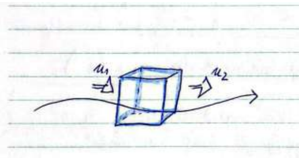
Slika 7.10: Skica k Lagrangeovski izpeljavi kontinuitetne enačbe.
