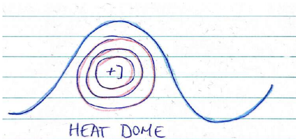
Slika 17.11: Stacionarno forsiranje Rossbyjevega vala z orografijo ali izvorom toplote.
