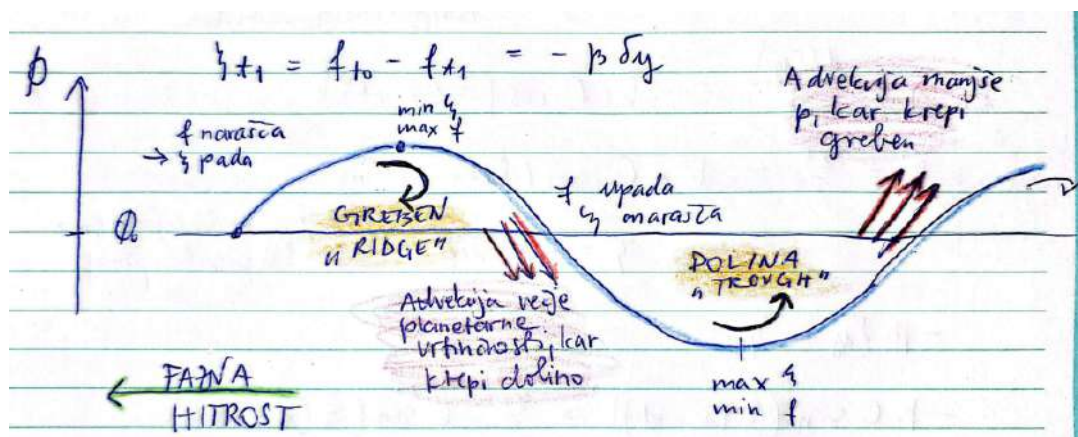
Slika 16.32: Skica ohranitve absolutne vrtničnosti pri meridionalnem odmiku delca.
