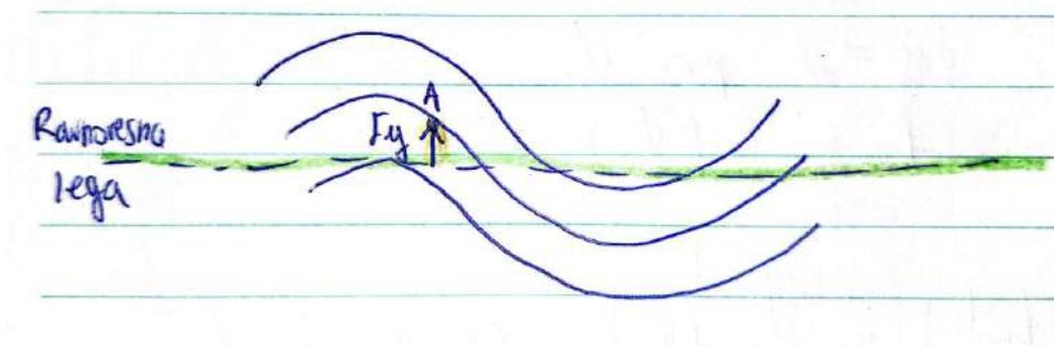
Slika 16.33: Idealiziran Rossbyjev val z oscilacijo v meridionalni smeri.
