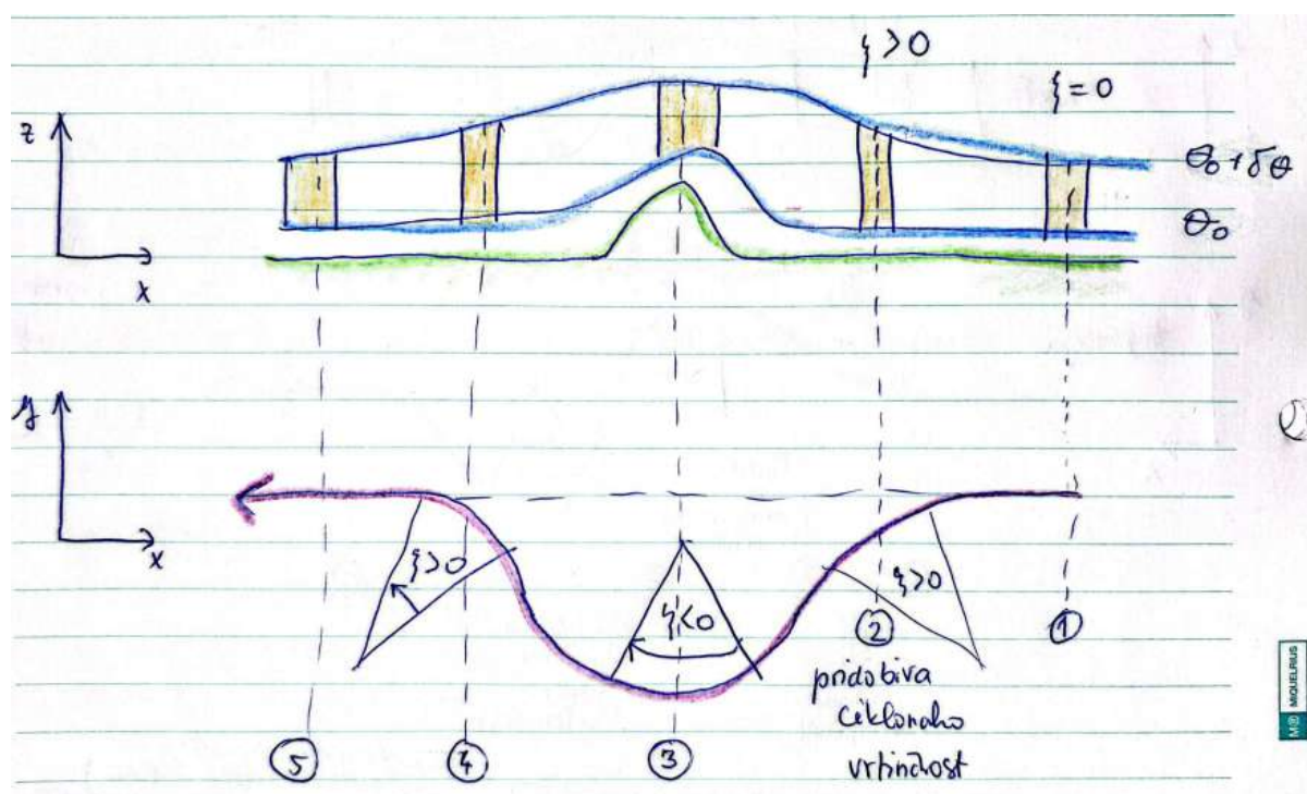
Slika 16.28: Vzhodni tok preko orografske ovire.
