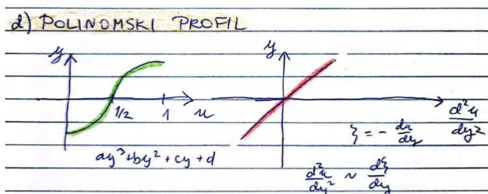
Slika 18.13: Skica drugega odvoda oziroma gradienta osnovne vrtinčnosti za polinomski profil. Na isti skici je prikazan tudi osnovni profil toka.
