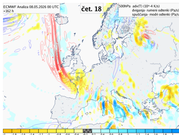
Slika 17.24: Primer lokalnega maksimuma tople advekcije južno od Irske. S tem je povezano območje dviganja, prikazano z rumenimi odtenki.
