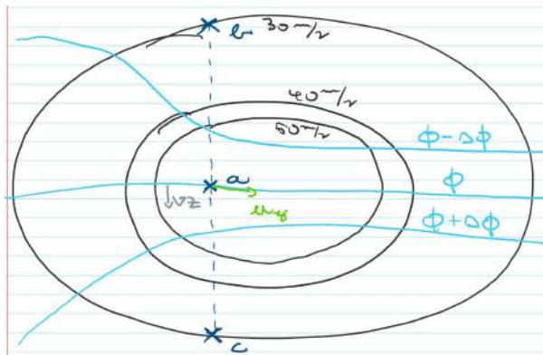
Slika 17.25: Skica konfluentnega zahodnega jet streama z izohipsami in izotahami.
