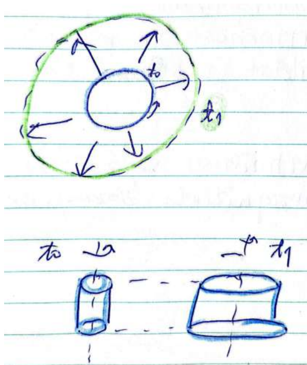
Slika 16.17: Ciklonalna vrtničnost: valj se ekspandira, a po drugi strani se vrtil počasneje.
