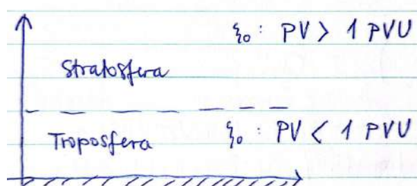
Slika 16.24: Vrednosti potencialne vrtinčnosti v troposferi in stratosferi.
