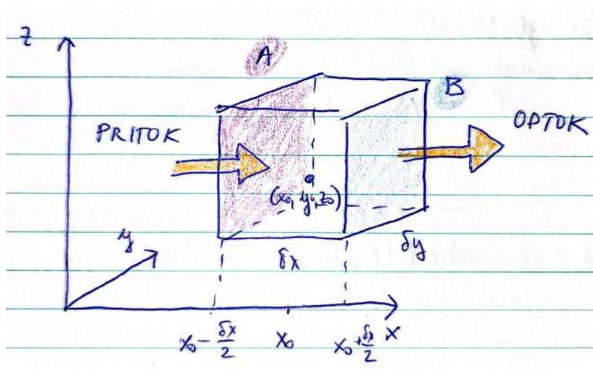
Slika 7.9: Kontrolni volumen za izpeljavo zakona o ohranitvi mase.
