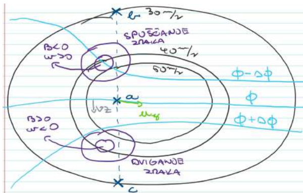
Slika 17.26: Presek skozi jet stream med hladnejšim in toplejšim stolpcem ter pripadajoča ageostrofska cirkulacija.
