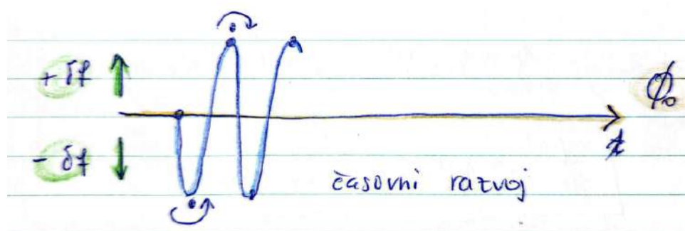
Slika 17.10: Mehanizem Rossbyjevega vala: odklon delca in izmenjava med planetarno ter relativno vrtničnostjo.
