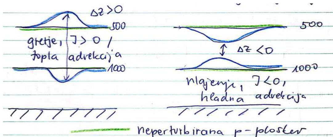
Slika 17.14: Vpliv diabatskega gretja in hlajenja na debelino plasti med izobarnima ploskvama. Levo je primer gretja, desno primer hlajenja.
