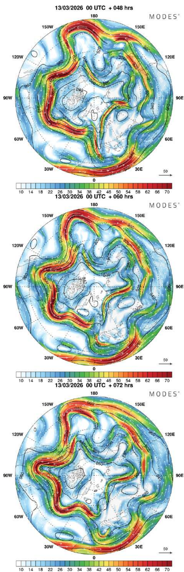
Slika 16.39: Dinamična meteorologija 150°W.
