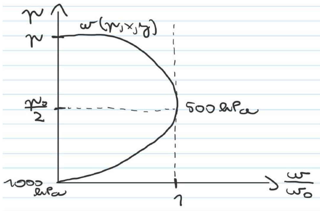
Slika 17.22: Idealiziran vertikalni profil \omega z maksimumom v srednji troposferi.
