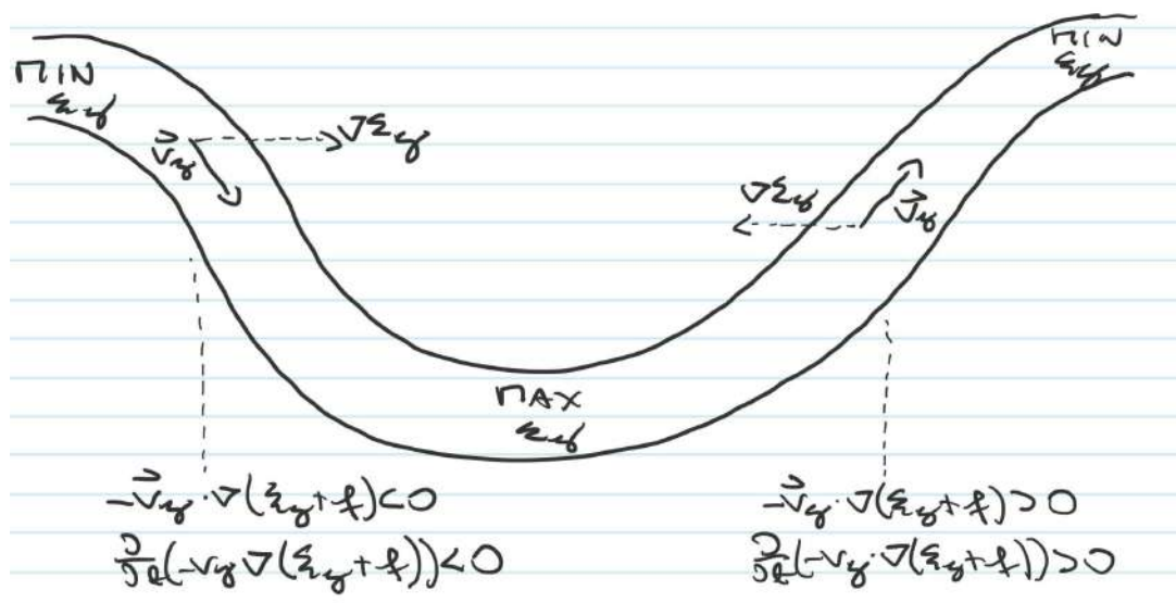
Slika 17.23: Skica Rossbyjevega vala z dolino, grebenom, geostrofskim vetrom in poljem relativne vrtničnosti.
