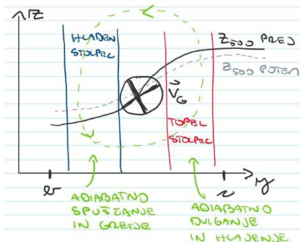
Slika 17.27: Razporeditev spuščanja in dviganja zraka ob jet streamu, ki pomaga obnoviti ravnovesje termalnega vetra.
