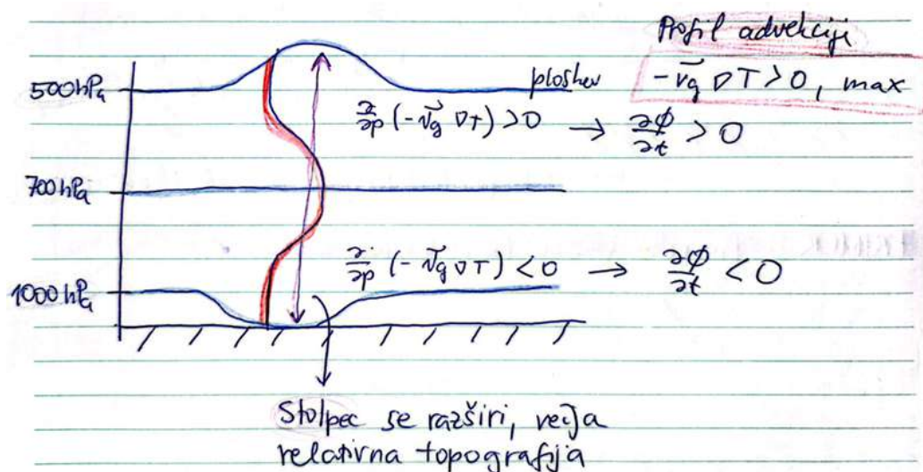
Slika 17.13: Skica vertikalnega profila tople advekcije z maksimumom v spodnji oziroma srednji troposferi.
