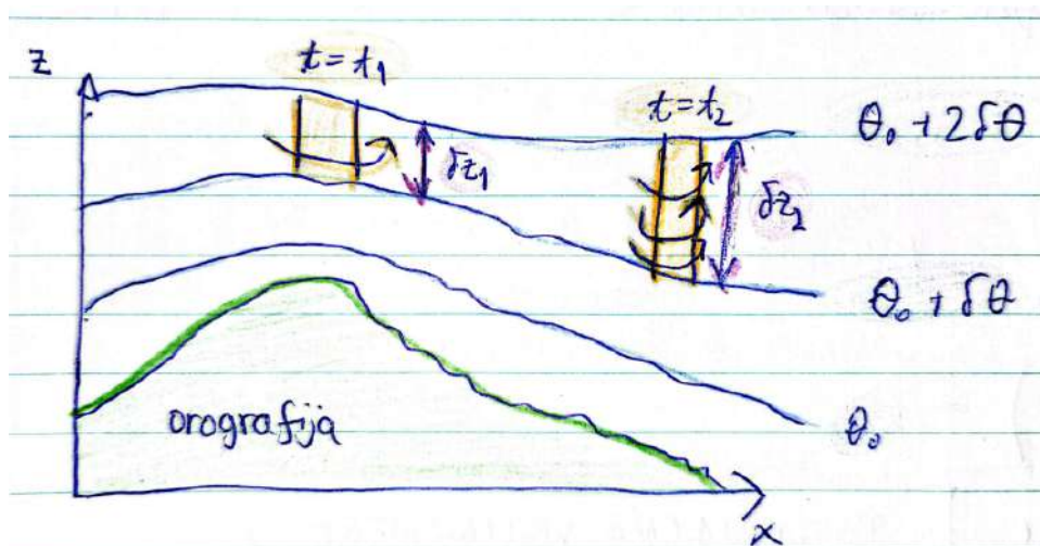
Slika 16.25: Skice za opis potencialne vrtinčnosti pri prehodu čez orografsko oviro.
