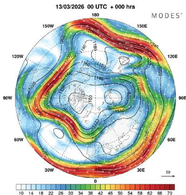
Slika 16.37: Tok na 200 hPa nad severno poloblo.
