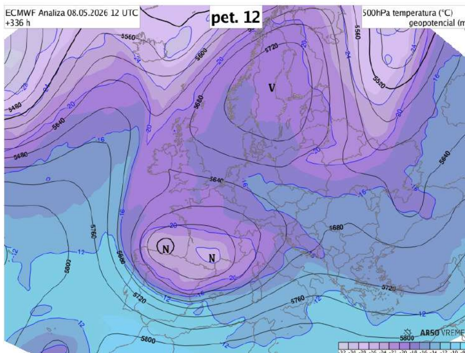
Slika 17.21: Odcepljeno jedro hladnega zraka nad Francijo in Španijo.
