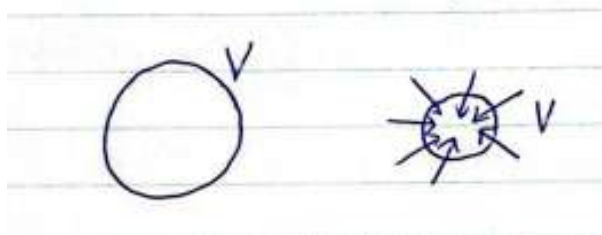
Slika 7.12: Pri divergenci se materialni volumen povečuje, pri konvergenci pa se skrči.
