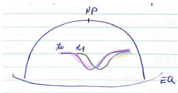
Slika 16.40: Skica kratkih valov.
