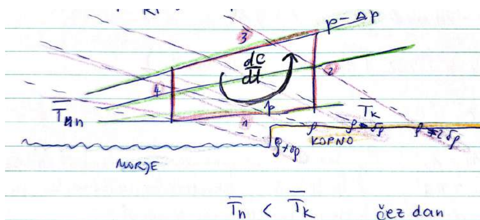
Slika 16.11: Skica cirkulacije na obali.
