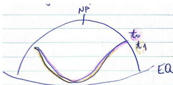
Slika 16.41: Skica dolgih valov.
