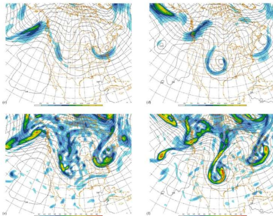
Slika 17.20: Primer močnejšega toka na zahodni oziroma gorvodni strani doline. S tem je skladno tudi polje vrtničnosti. Člen B v tem primeru deluje tako, da advektira pozitivno vrtničnost, zato je B > 0 . Vrtničnost v dolini se poveča, dobimo \frac{\partial \Phi}{\partial t} < 0 , dolina se poglobi, hkrati pa se translira proti ekvatorju.
