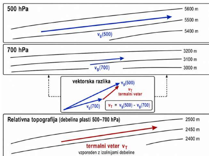
Slika 15.7: Skica geostrofskega vetra na dveh različnih višinah in pomen termalnega vetra v tem primeru.
