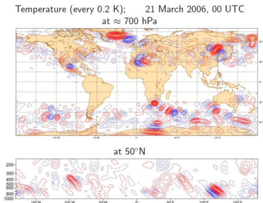
Slika 9.16: Temperaturne motnje, povezane z vodilnim singularni vektorji pri 700 hPa (zgoraj) in navpičnici prečni prerez vzdolž 50^\circ\text{N} (spodaj). Pojavijo se maksimumi nad sledovi neviht na južni polobli in Islandiji minimum, tj. v dinamično aktivnih regijah z velikimi rast napake napovedi.
