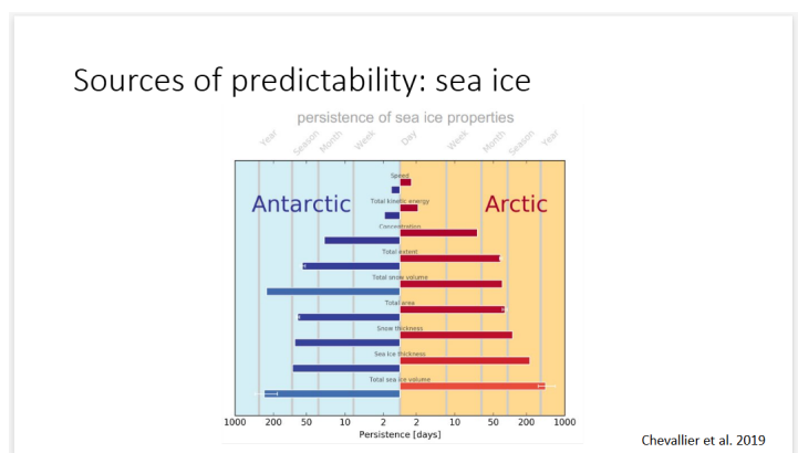
Slika 8.23: Vztrajnost spremenljivk morskega ledu. Vrstice prikazujejo čas zvijanja, dokler avtokorelacija ne pade pod e^{-1} . Modra = Antarktika; rdeča = Arktika.
