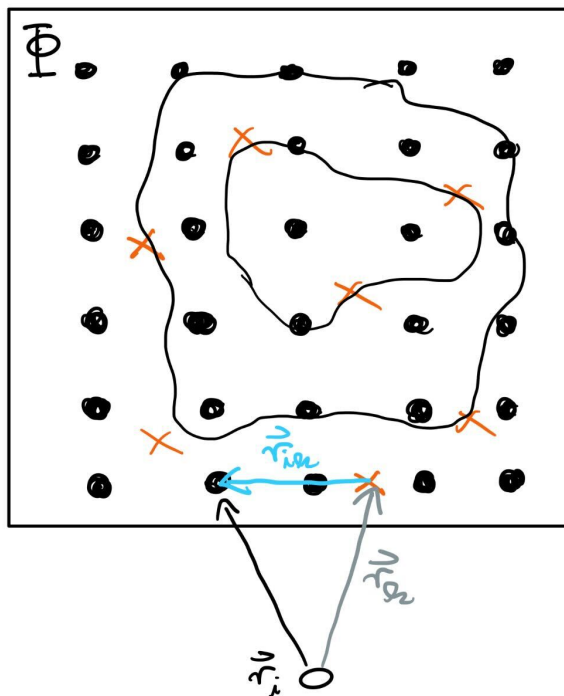
Slika 2.4: Shematski prikaz metode zaporednega korigiranja. Črne pike ( \bullet ) označujejo modelne mrežne točke \vec{r}_i , oranžni križci ( \times ) pa lokacije meritev \vec{r}_k . Črne krivulje lahko ponazarjajo izolinijske ozadnega polja. Puščice nakazujejo, kako meritve na lokaciji \vec{r}_k vplivajo na analizo v bližnji mrežni točki \vec{r}_i .
