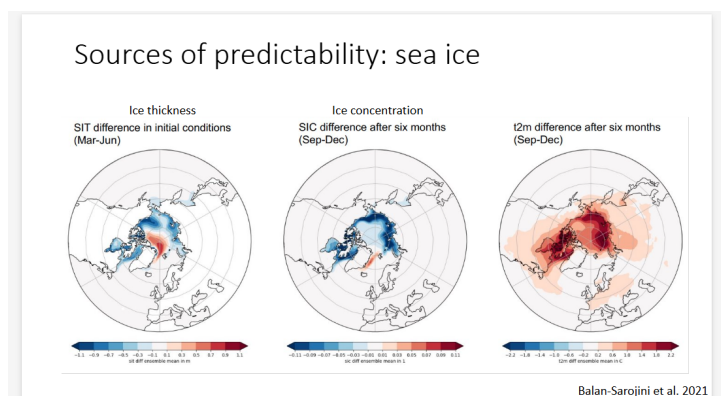
Slika 8.22: Ensemble-mean občutljivost na 1m motnjo debeline arktičnega morskega ledu (SIT) v marcu–juniju (levo). Odzivi september–december: koncentracija morskega ledu (na sredini) in temperatura 2 m (desno). Modra = hladnejše, rdeča = toplejša. (Balan-Sarajini et al. 2021)
