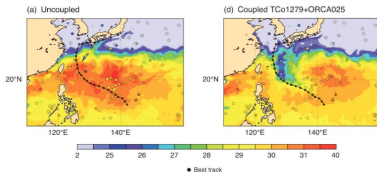
Slika 8.20: Petdnevna napoved SST med tajfunom Haiyan. Levo: nepovezana atmosfera. Desno: spoj atmosfera–ocean na 25km. Sklapanje zajame hladno sled in izboljša predvidevanje sledi/intenzivnosti.
