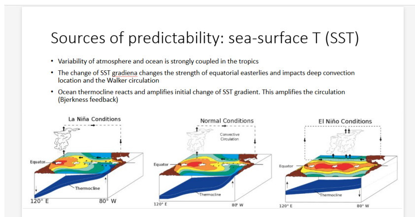
Slika 8.18: Skica Bjerknesove povratne informacije: gradient SST \Rightarrow anomalija vzhodnega vetra \Rightarrow nagib termoklina \Rightarrow povečan gradient SST. Plošče prikazujejo La Niña, nevtralna stanja in El Niño.
