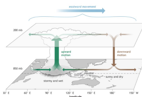
Slika 8.17: Konceptualni model konvektivne ovojnice MJO, ki se širi proti vzhodu. Zelene puščice: naraščajoča veja; rjave puščice: posedanje.
