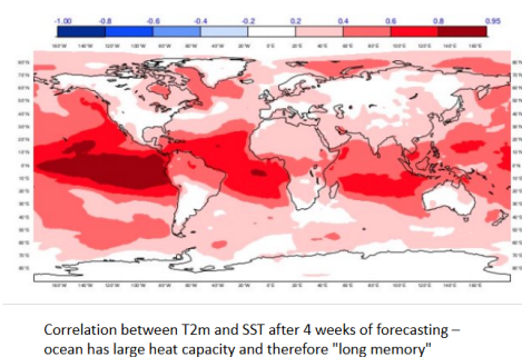
Slika 8.19: Korelacija štiritedenskih anomalij napovedi T_{2m} z začetnim SST. Rdeča območja označujejo močan oceanski nadzor.
