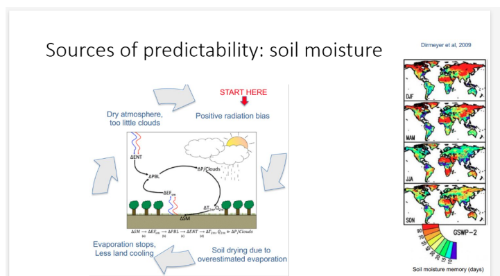
Slika 8.21: Povratna zanka zemlja-atmosfera. Pozitivno sevanje izsuši zemljo, zmanjša latentni toplotni tok, zviša T_{2m} in dodatno izsuši zemljo.
