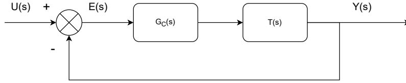
Figure 6: Sistema com Controlador.
