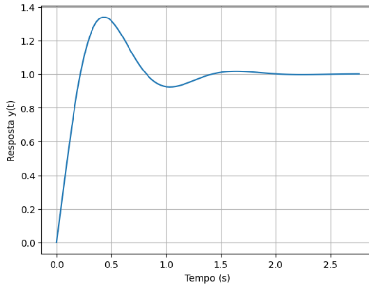
Figure 7: Resposta ao degrau sem controlador.
