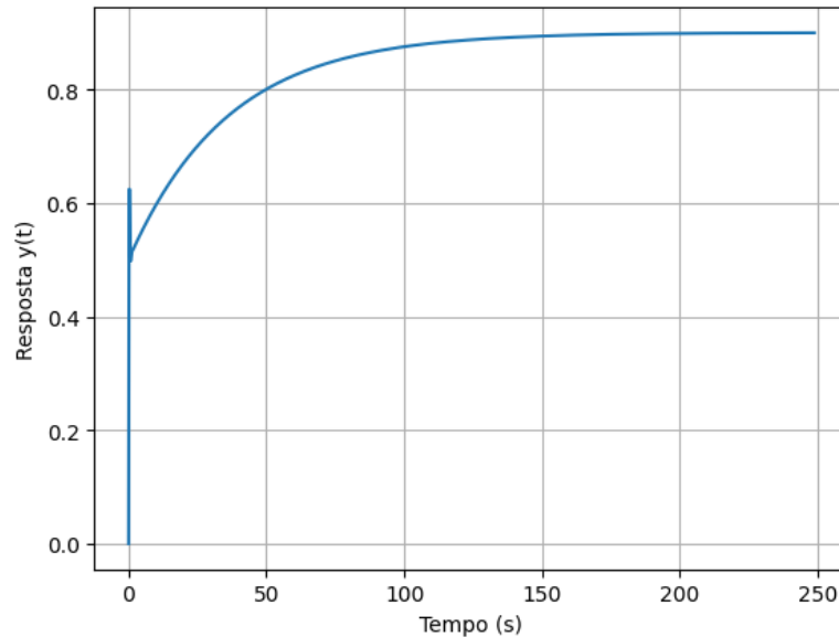
Figure 8: Resposta ao degrau com controlador.
