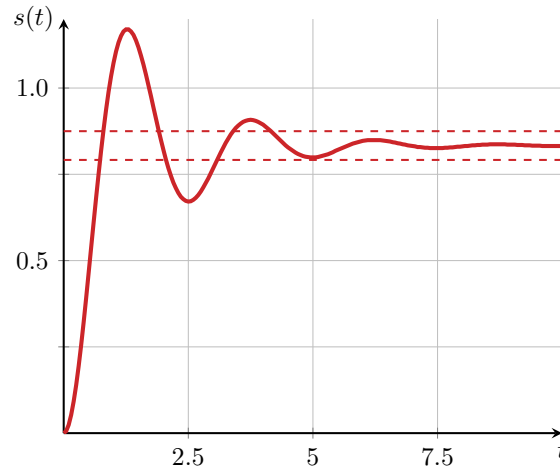
Figure 8.4 – Réponse indicielle du système en boucle fermée non corrigé
