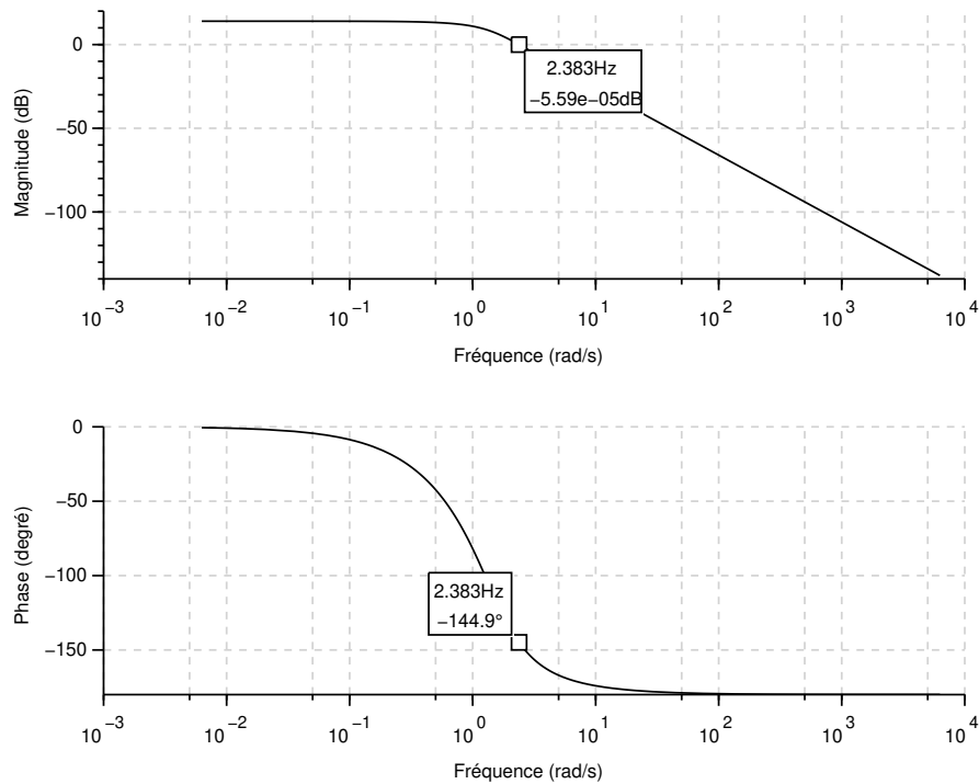
Figure 8.2 – Diagramme de Bode de la boucle ouverte non corrigée. On a représenté le gain et la phase à la pulsation de coupure \omega_{0\text{dB}} du système non corrigée.
