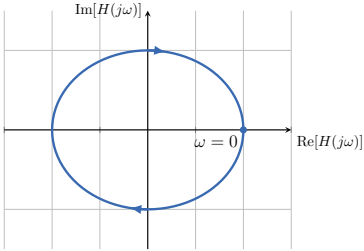
FIGURE 4.21 : Diagramme de Nyquist d'un retard pur. Le lieu de Nyquist est représenté par le cercle unité dans le plan complexe.
