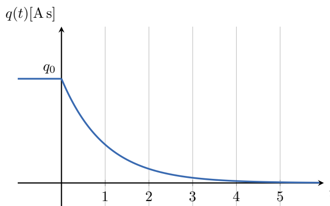
Figure 1.15 – Charge aux bornes du condensateur en fonction du temps.
