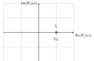
FIGURE 4.18 : Diagramme de Nyquist d'un gain pur. Le nombre complexe H(j\omega) est représenté par un point sur l'axe des réels à la valeur K .
