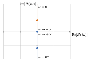
FIGURE 4.19 : Diagramme de Nyquist d'un intégrateur pur. Le lieu de Nyquist est représenté par une demi droite sur l'axe des nombres imaginaires purs négatifs.
