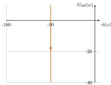
FIGURE 4.25 : Diagramme de Black d'un intégrateur pur. Le lieu de Black est représenté par une droite d'abscisse -90^\circ .
