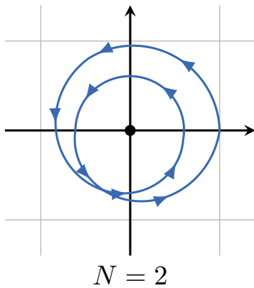
FIGURE 7.11 : Représentation schématique du nombre de tours N autour de l'origine de l'image d'une fraction rationnelle d'un contour fermé. Le sens positif est celui du sens trigonométrique.
