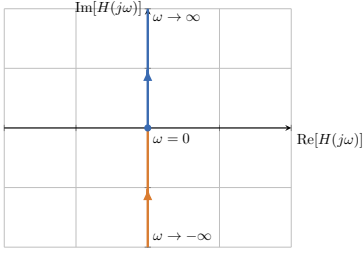
FIGURE 4.20 : Diagramme de Nyquist d'un dérivateur pur. Le lieu de Nyquist est représenté par une demi-droite sur l'axe des nombres imaginaires purs positifs.
