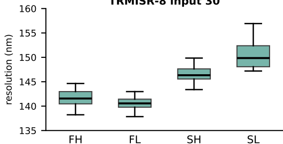
TRMISR-8 input 30
