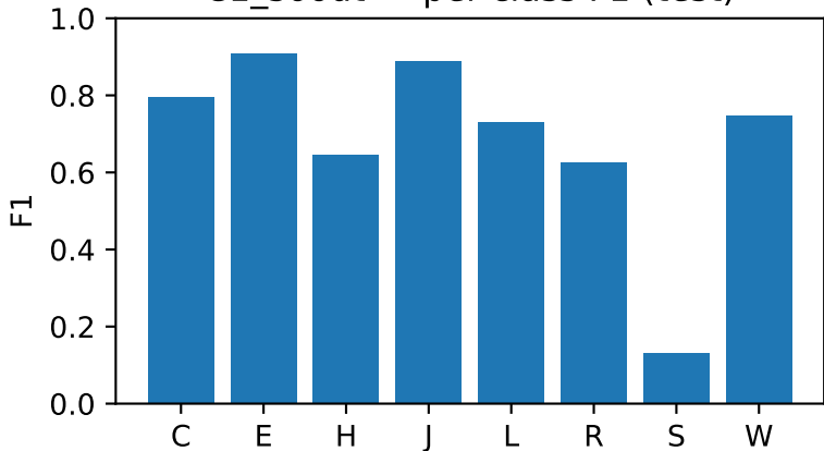
C1_s6out — per-class F1 (test)
