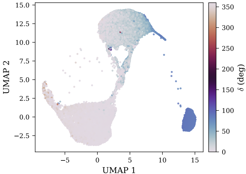
UMAP embedding
