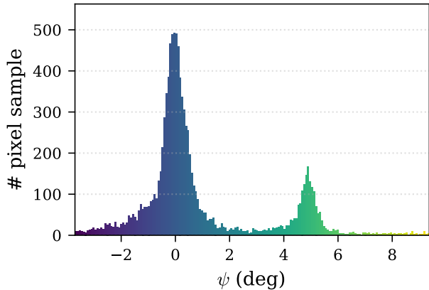
Istogramma \psi
