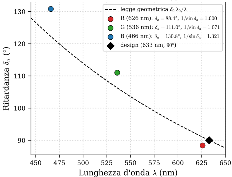
Calibrazione di \delta_a : misura vs legge 1/\lambda
