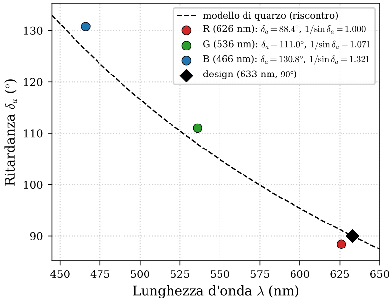
Calibrazione di \delta_a : misura vs modello di quarzo
