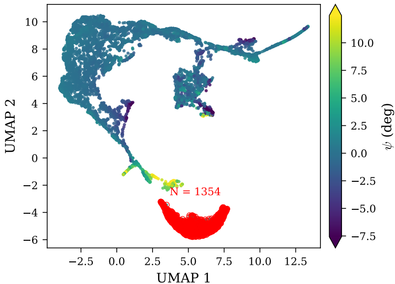
UMAP embedding
