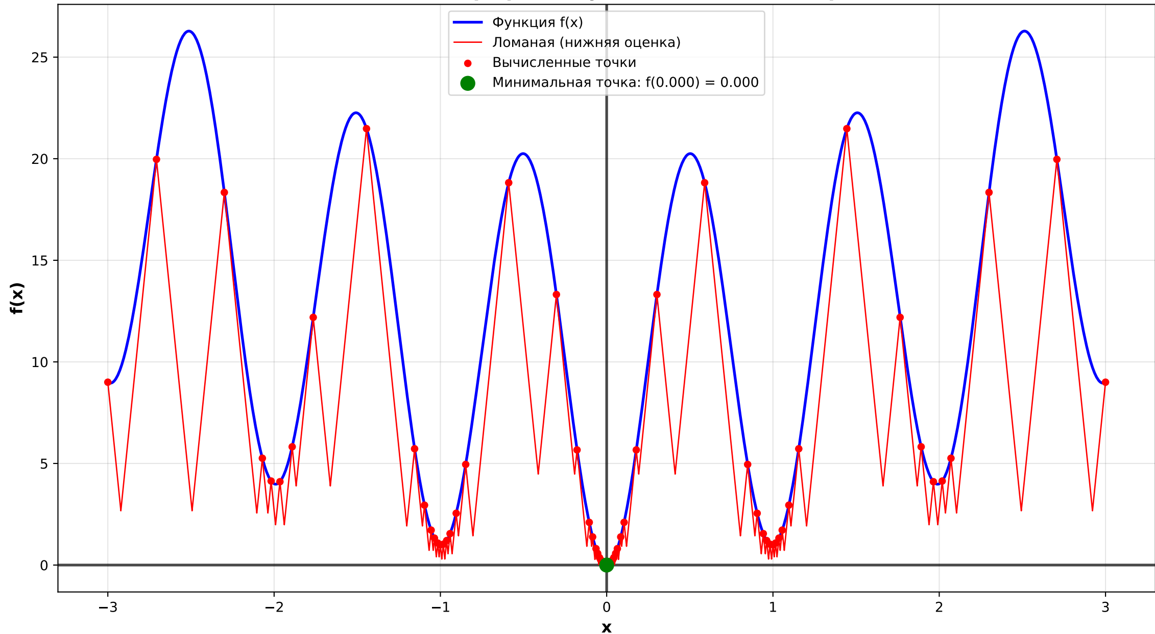
Метод Пиявского - График текущего состояния (итерация #176)
