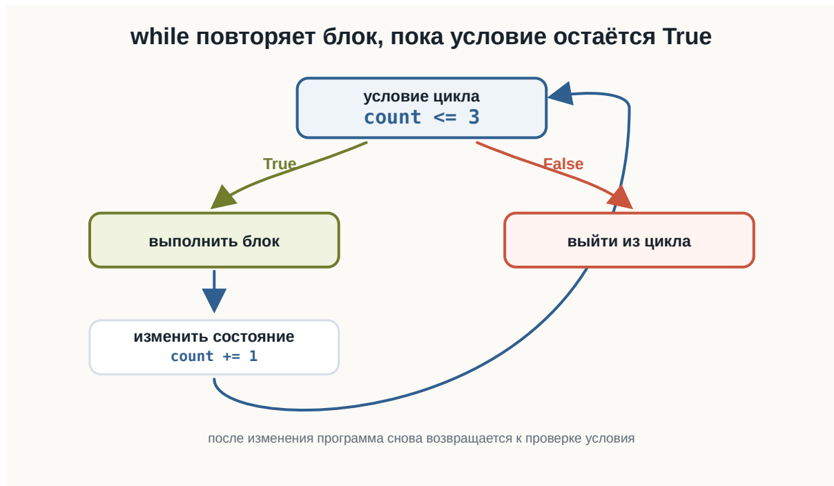
Рисунок 2.66: Схема работы цикла while
