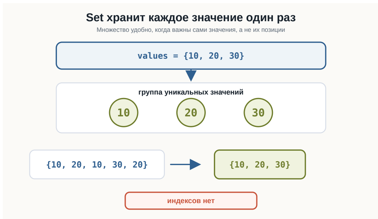
Рисунок 2.96: Устройство множества
