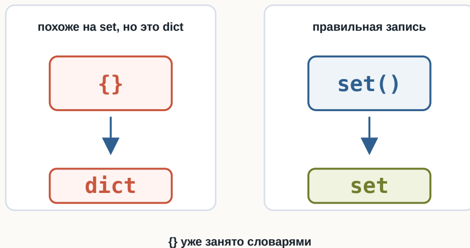
Рисунок 2.97: Пустое множество
