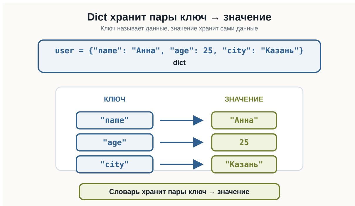
Рисунок 2.101: Устройство словаря
