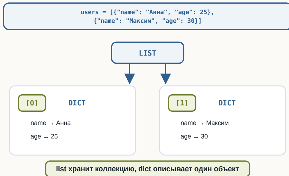
Рисунок 2.111: Список словарей
