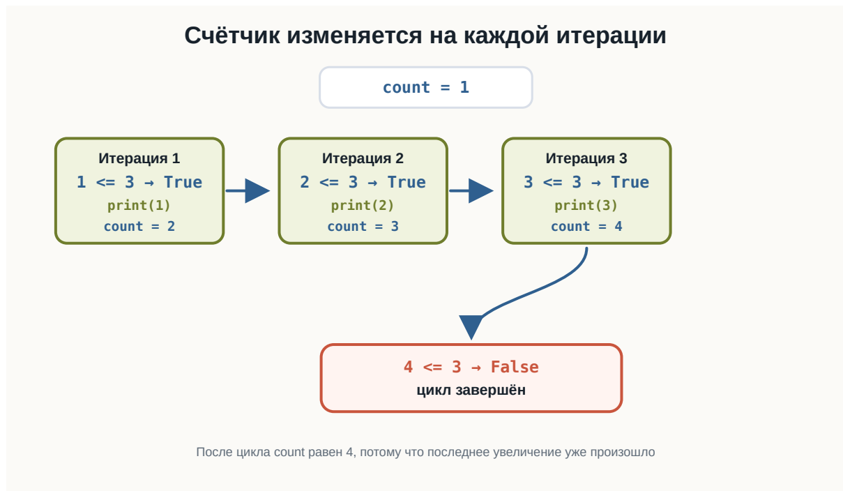
Рисунок 2.67: Пошаговое изменение счётчика в while
