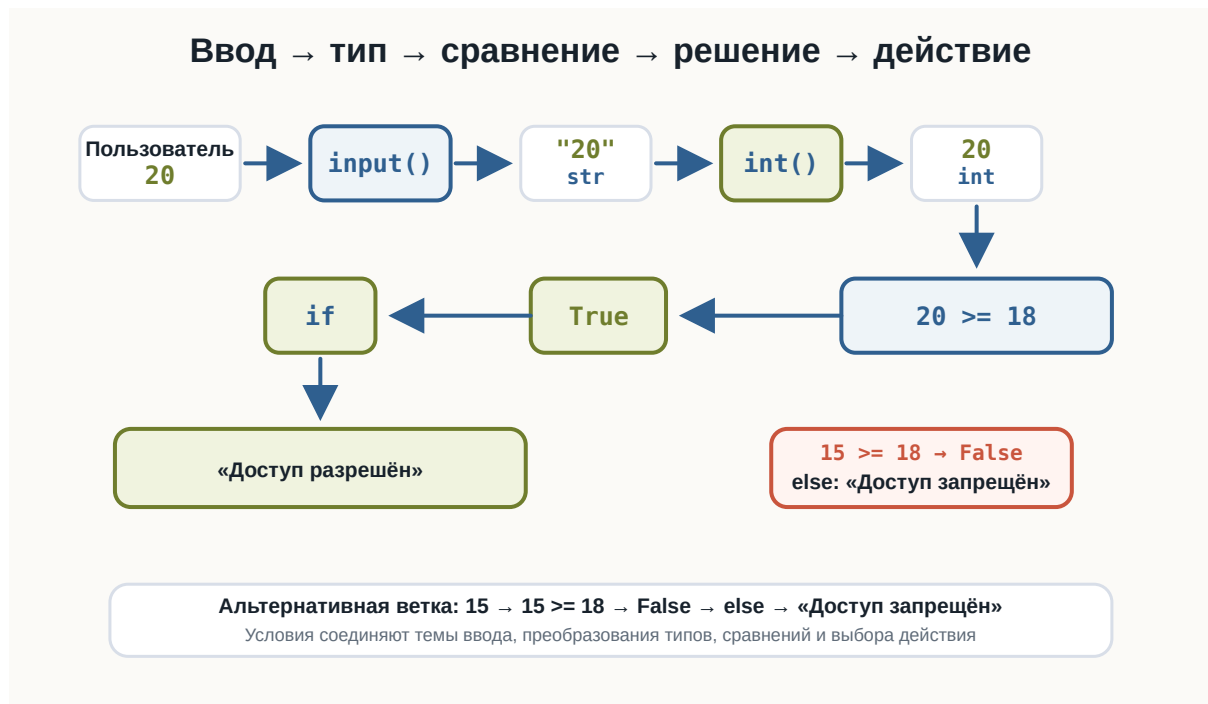
Рисунок 1.58: Ввод, преобразование типа, сравнение и решение
