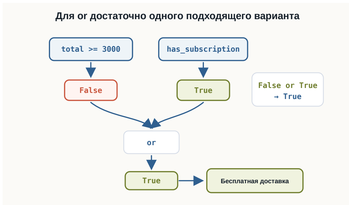
Рисунок 1.63: Поток решения для оператора or
