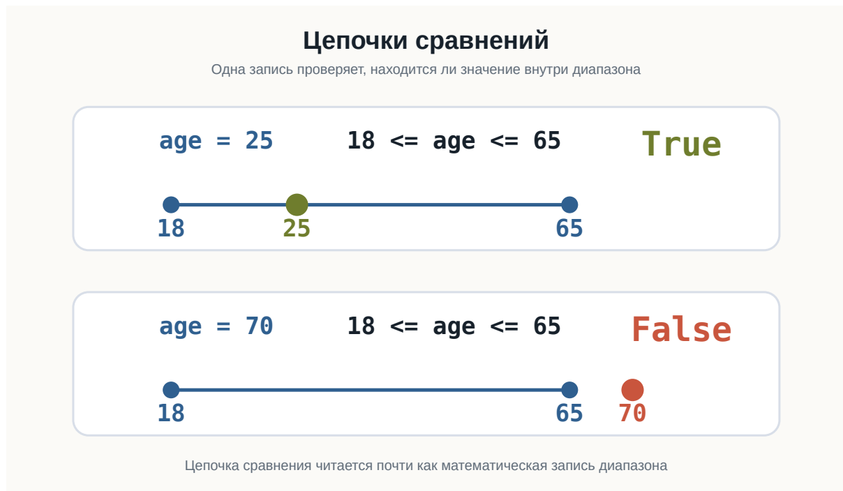
Рисунок 1.55: Цепочка сравнений проверяет диапазон
