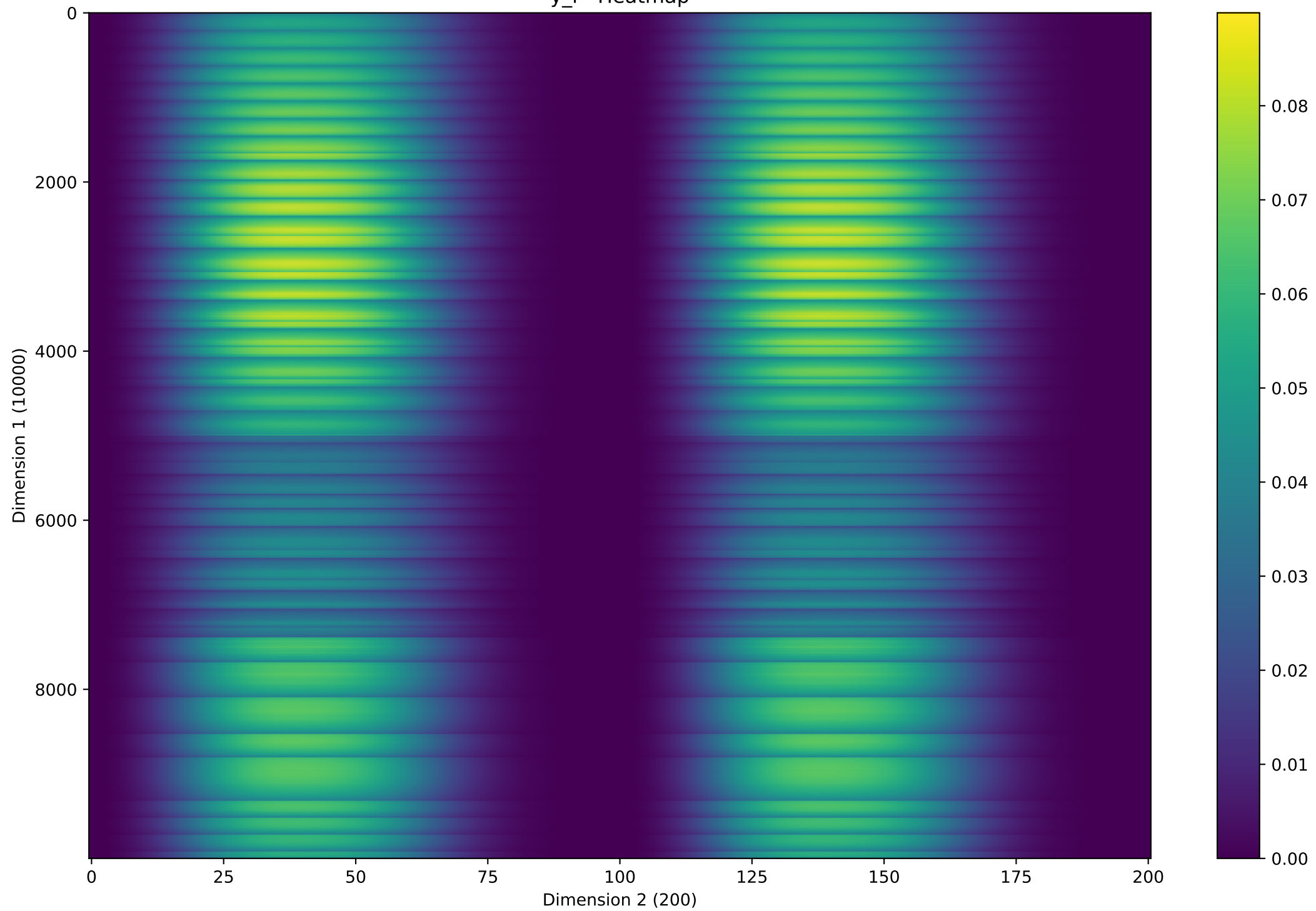
y_l - Heatmap
