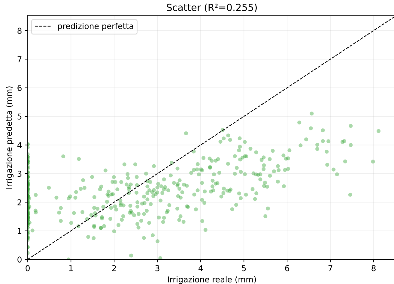
Fig. 2 — Predicted vs actual, LSTM (miglior modello), H=1, test set 2020-2022
