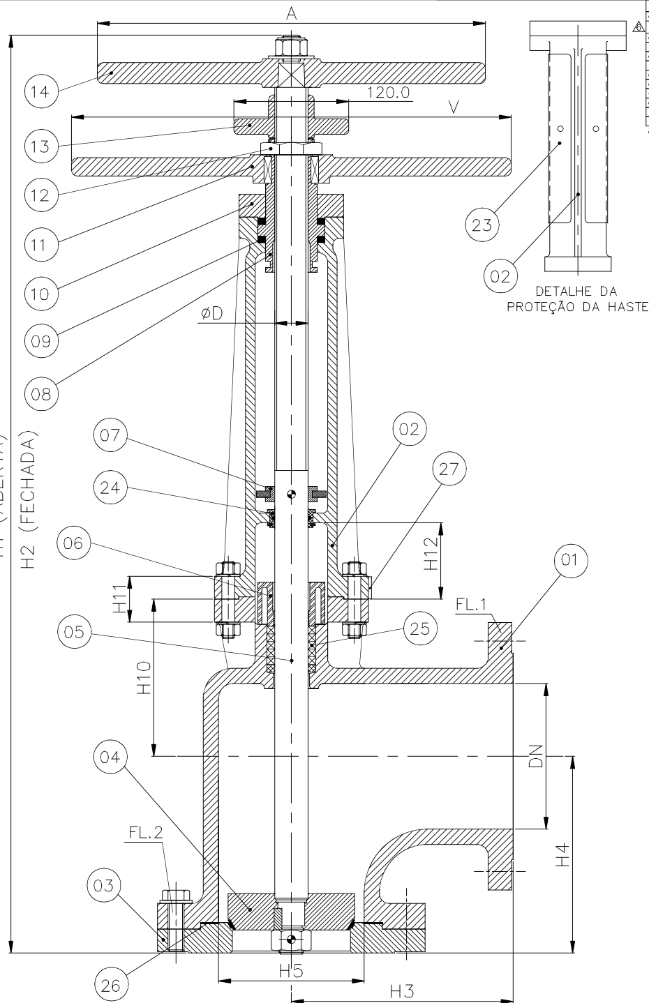
MONTAGEM C/ VOLANTE MANUAL (VALVULA AS1)
