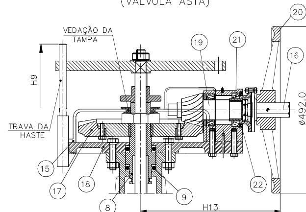
MONTAGEM C/ ATUADOR (VALVULA AS1A)
