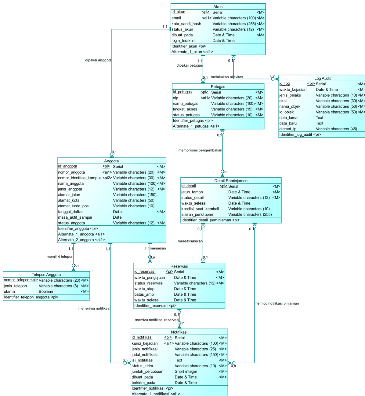
Gambar 5.5: CDM bagian akun, notifikasi, dan audit
