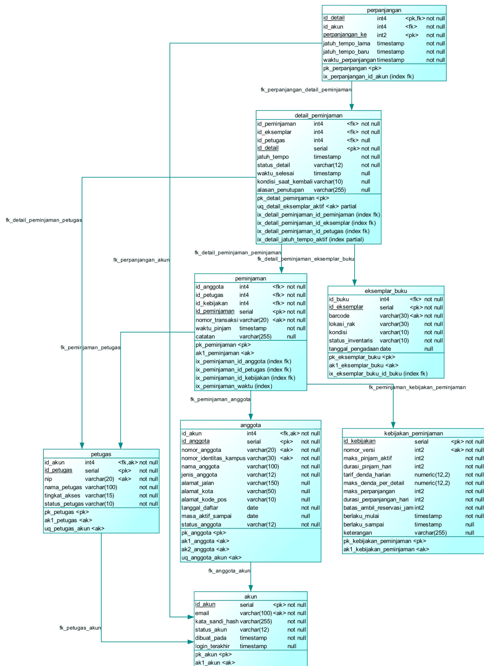
Gambar 7.4: PDM bagian peminjaman dan perpanjangan
