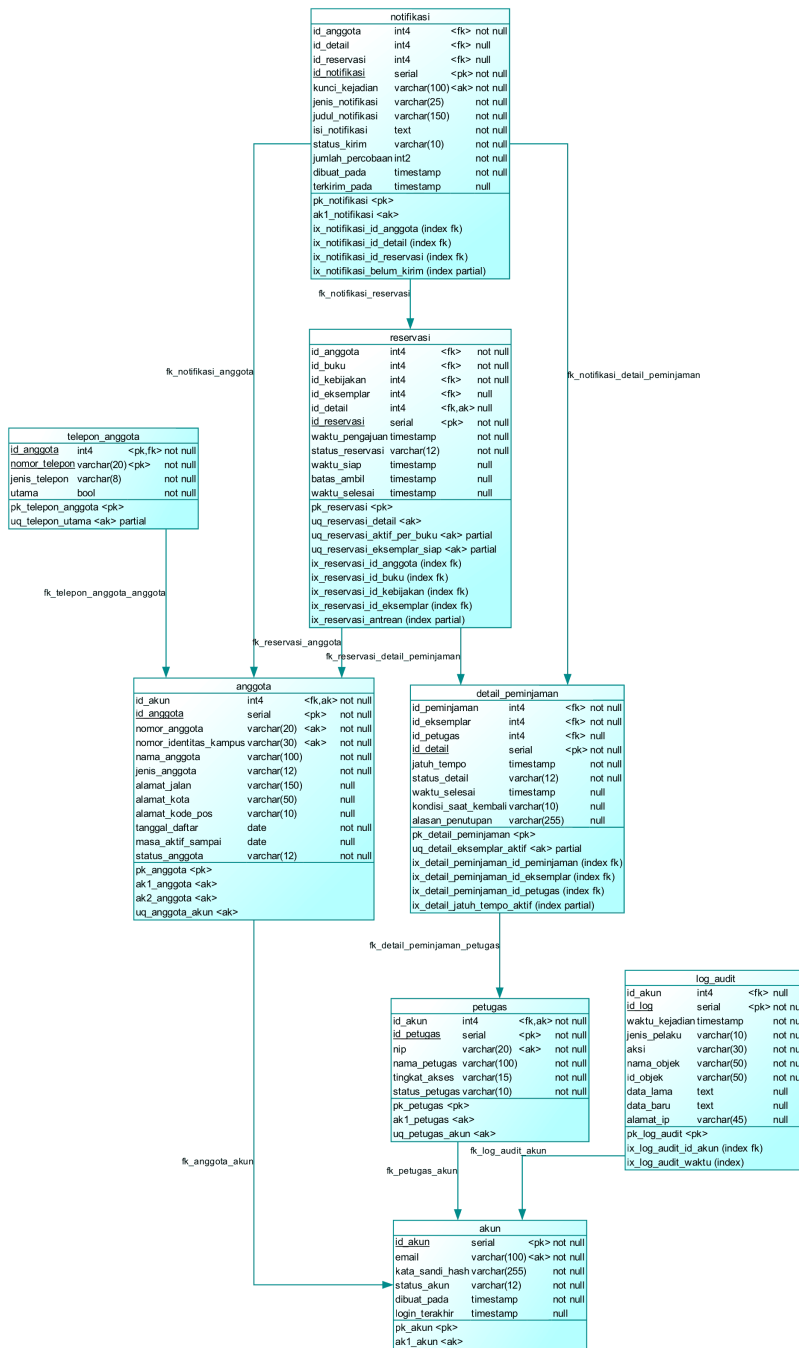
Gambar 7.6: PDM bagian akun, notifikasi, dan audit
