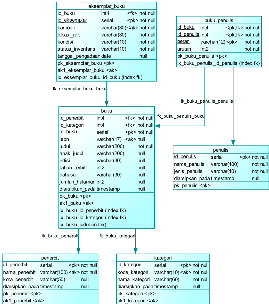
Gambar 7.3: PDM bagian katalog dan salinan fisik
