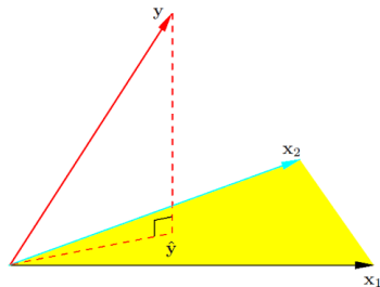
图 1: 线性回归的几何视角
