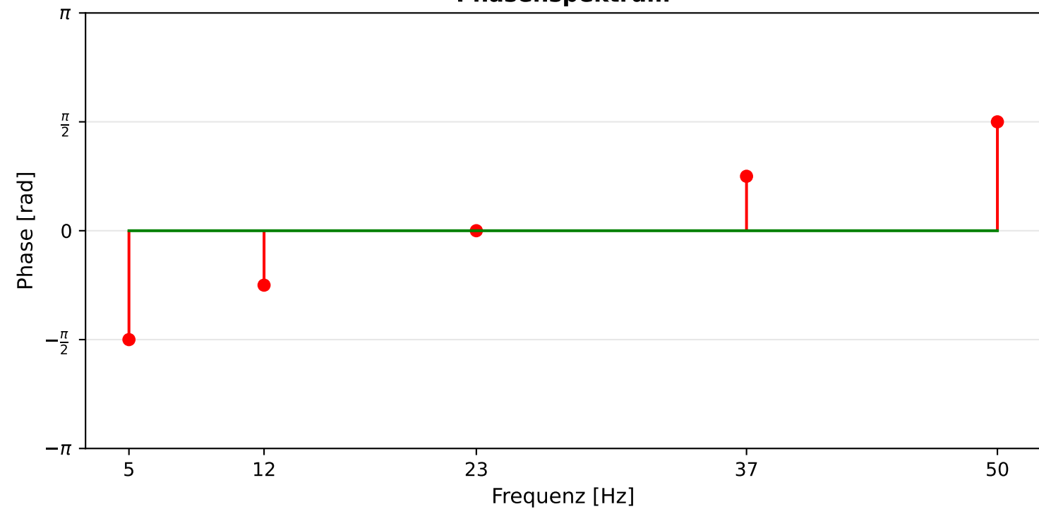
Phasenspektrum
