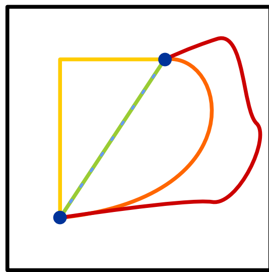
Euklidische Norm im \mathbb{R}^2
