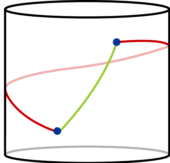
Metrik auf dem Zylinder
