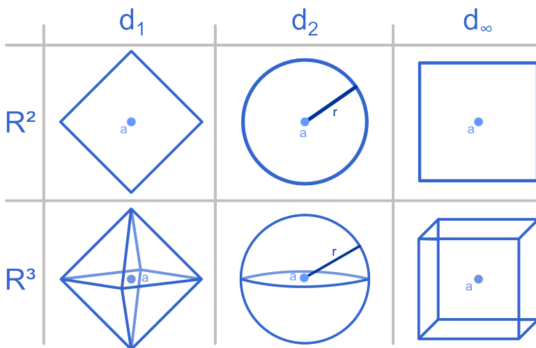
Figure 2: Einheitsbälle im \mathbb{R}^2 und \mathbb{R}^3 für die Normen d_1, d_2, d_\infty
