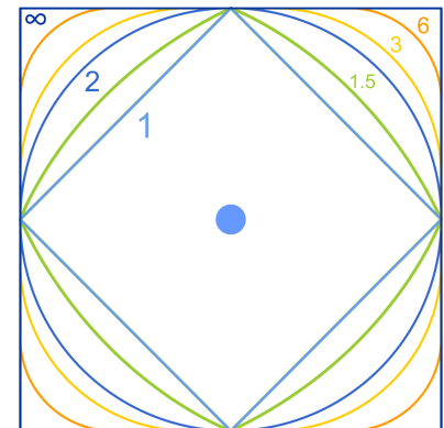
Figure 3: Beispielhafte "Entwicklung" von Einheitsbällen verschiedener Normen
