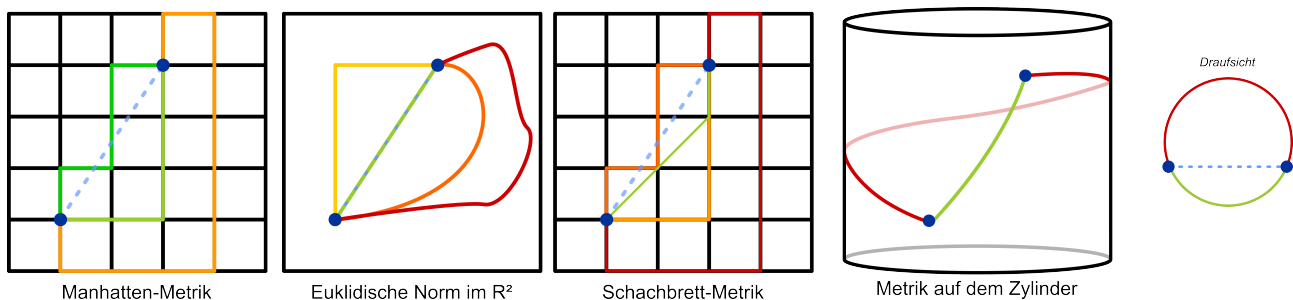
Figure 1: Bekannte metrische Räume
