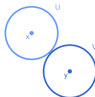
Abb. ?? : Visualisierung Hausdorff-Raum
