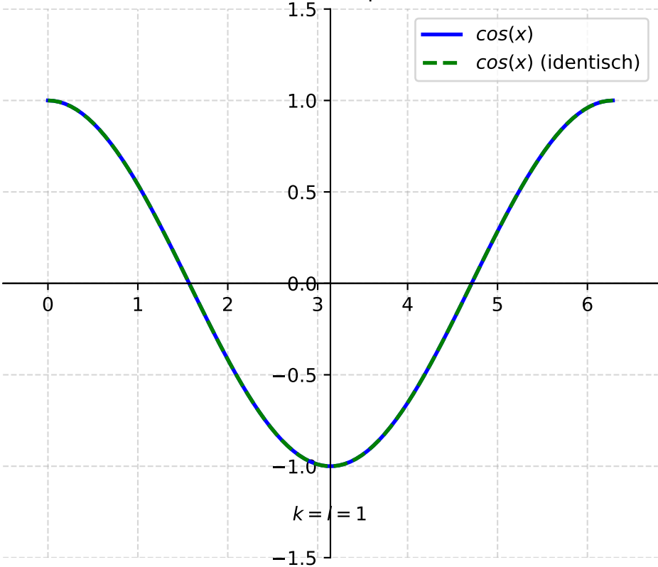
\cos(kx), \cos(lx) \mid l = k \neq 0
