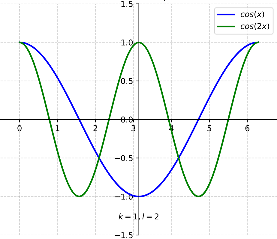
\cos(kx), \cos(lx) \mid l \neq k
