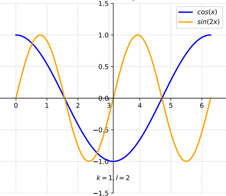
\cos(kx), \sin(lx) \mid l \neq k
