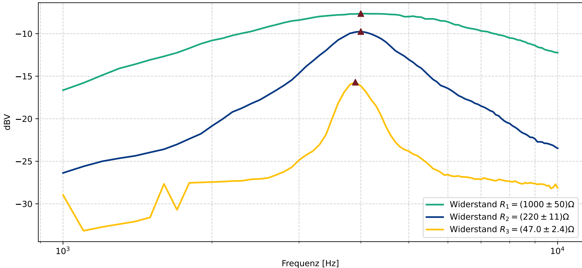
Frequenzgang mit Maxima
