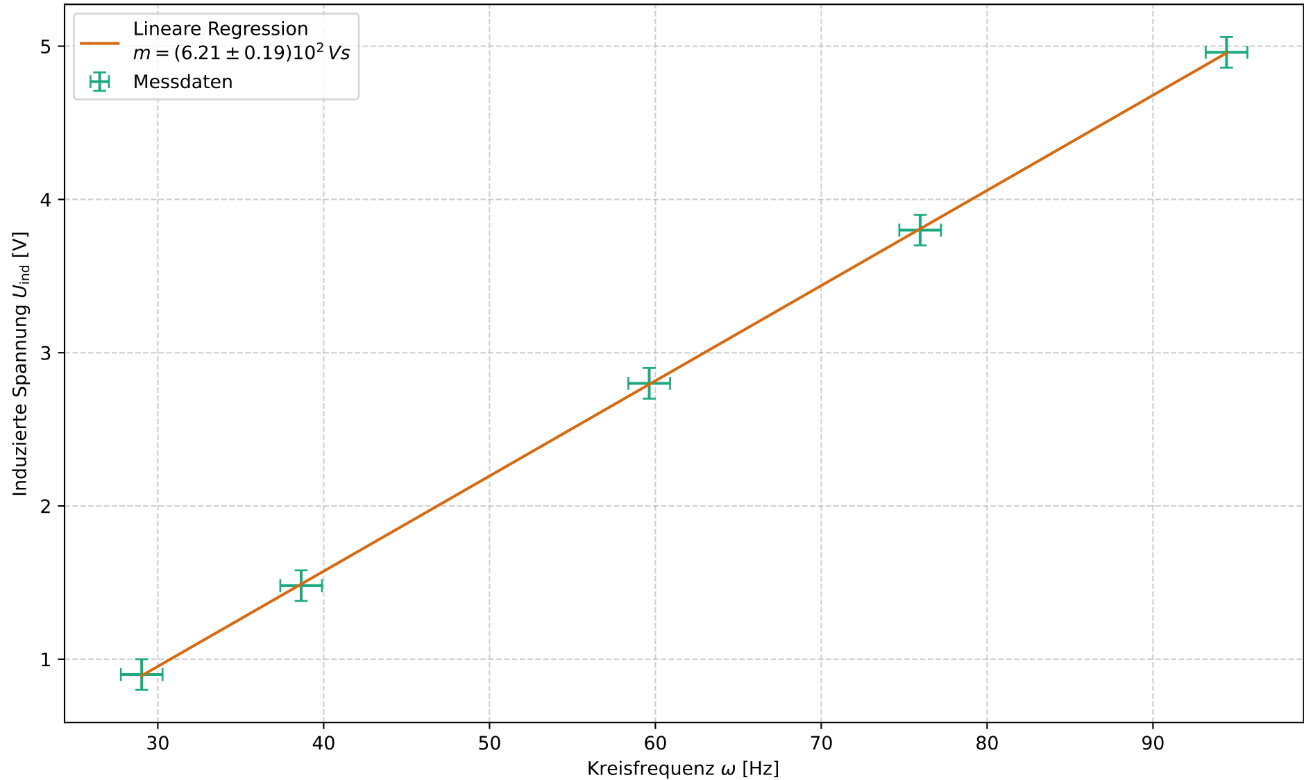
Induktionsspannung in Abhängigkeit der Frequenz
