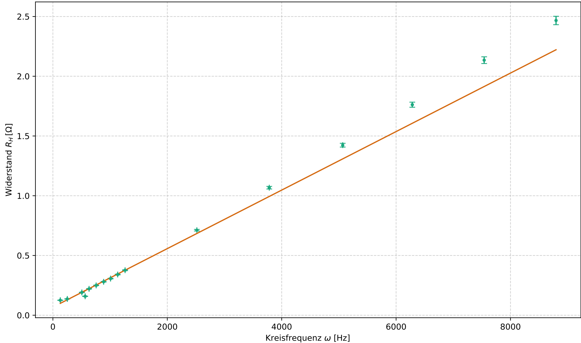
Widerstand in der Helmholtzspule
