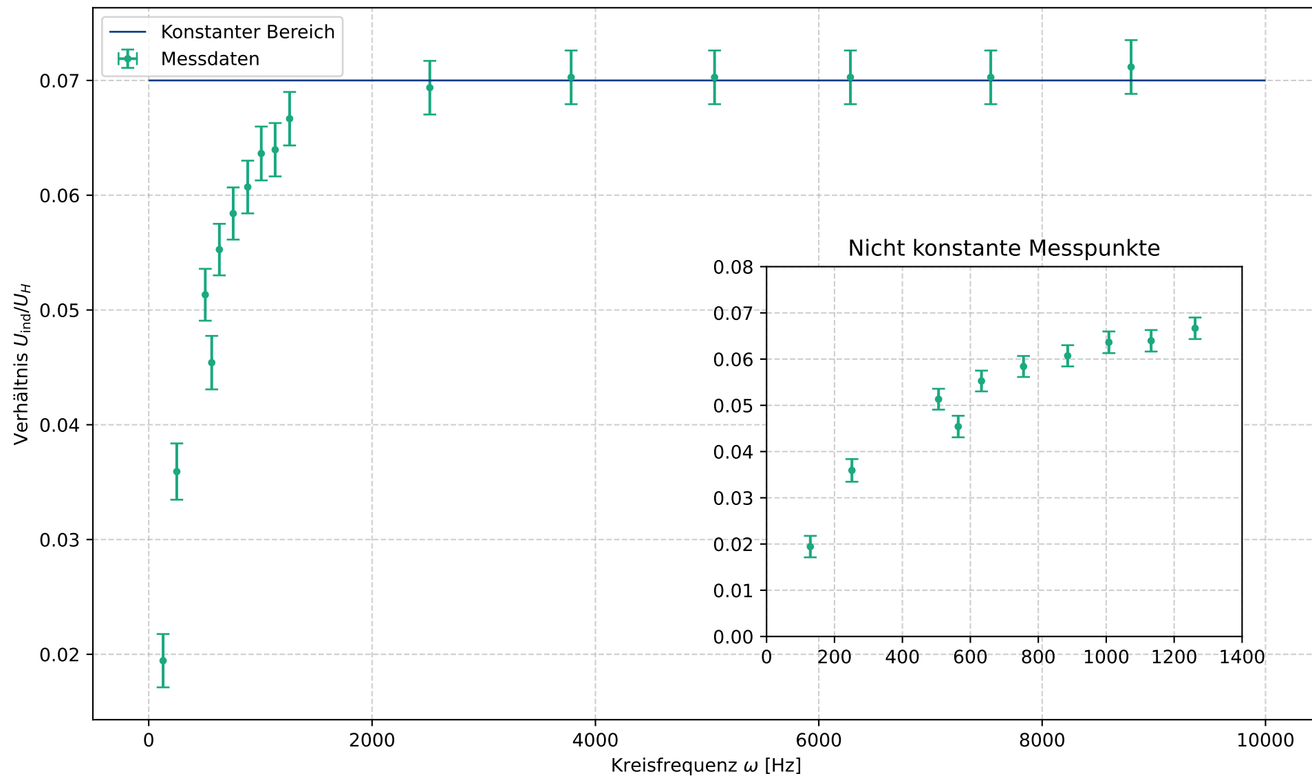
Kennlinie des Lufttransformators
