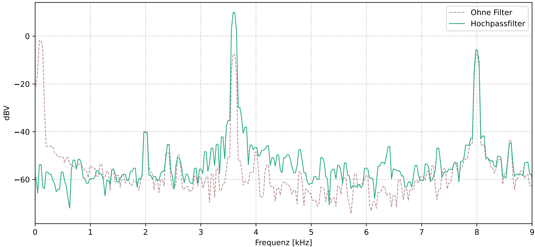
FFT Vergleich: Hochpass vs. Ohne Filter
