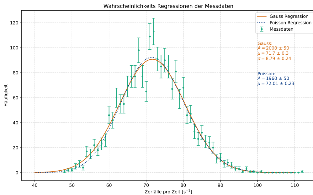
Abbildung 4.II: Messdaten mit Regressionsfunktionen: Gauss- und Poissonverteilungen.
