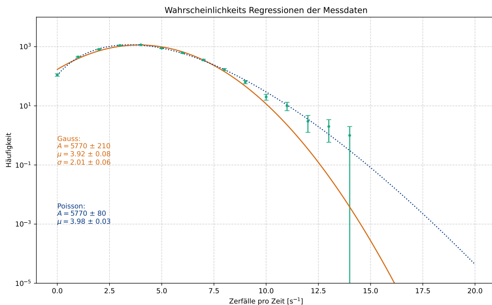
Abbildung 4.III: Messdaten mit Regressionsfunktionen: Gauss- und Poissonverteilungen.
