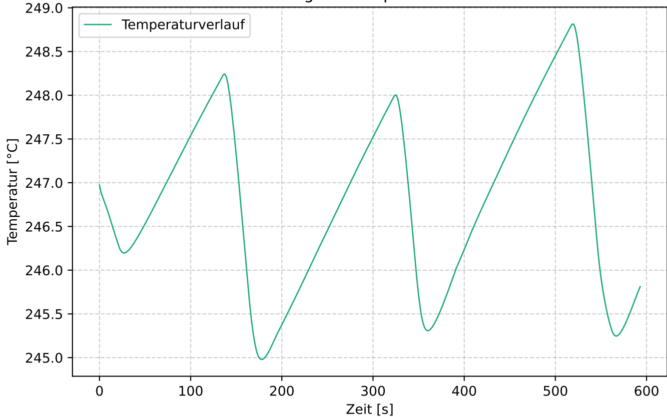
Schwankung der Temperatur bei 250°C
