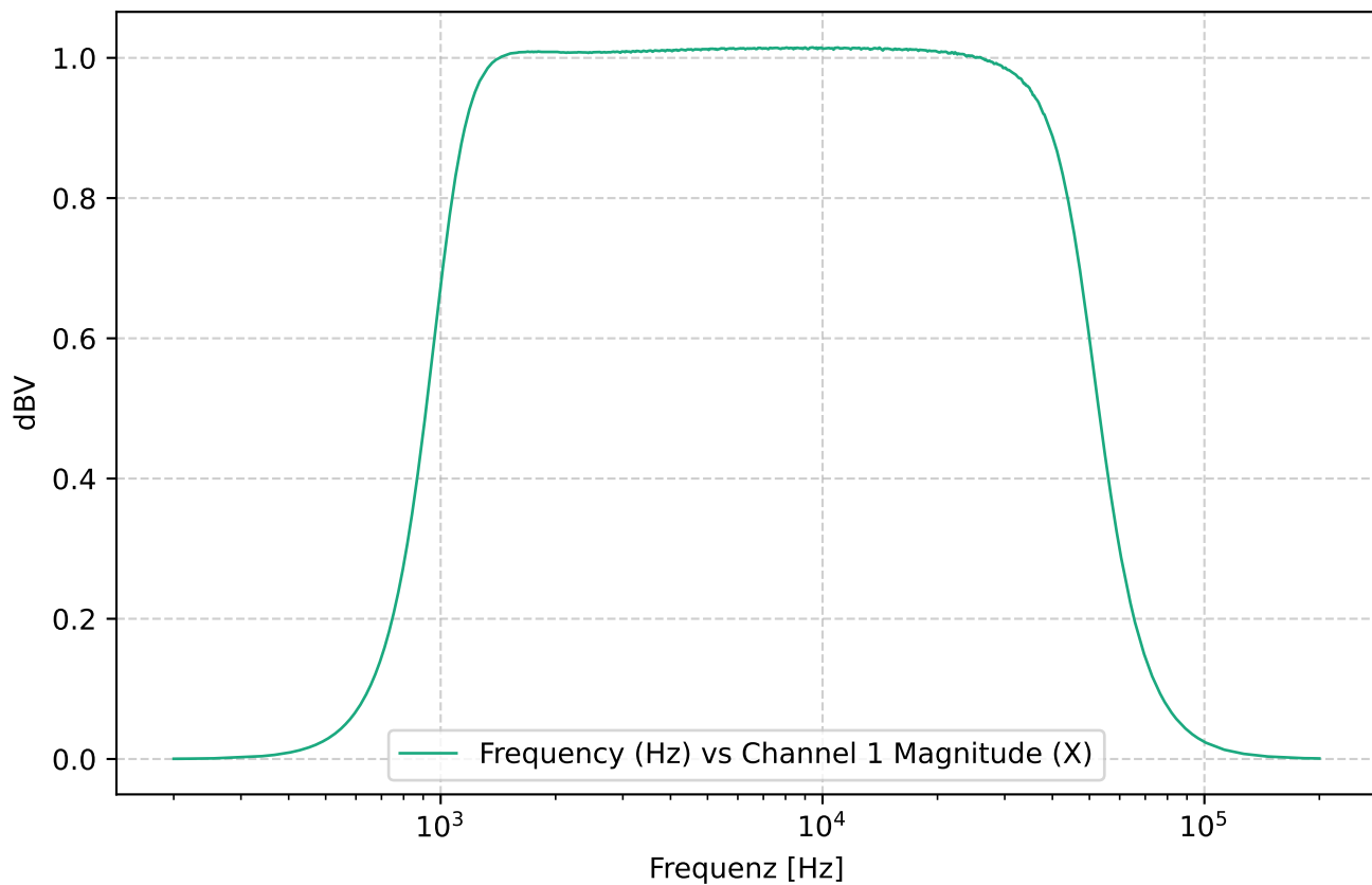
Frequenzgang mit Bandpassfilter (5k \Omega )
