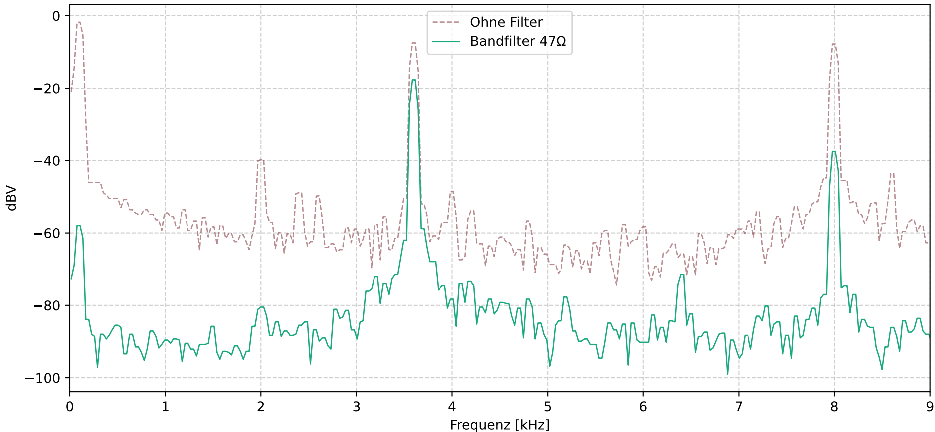
FFT Vergleich: 47 Ohm vs. Ohne Filter
