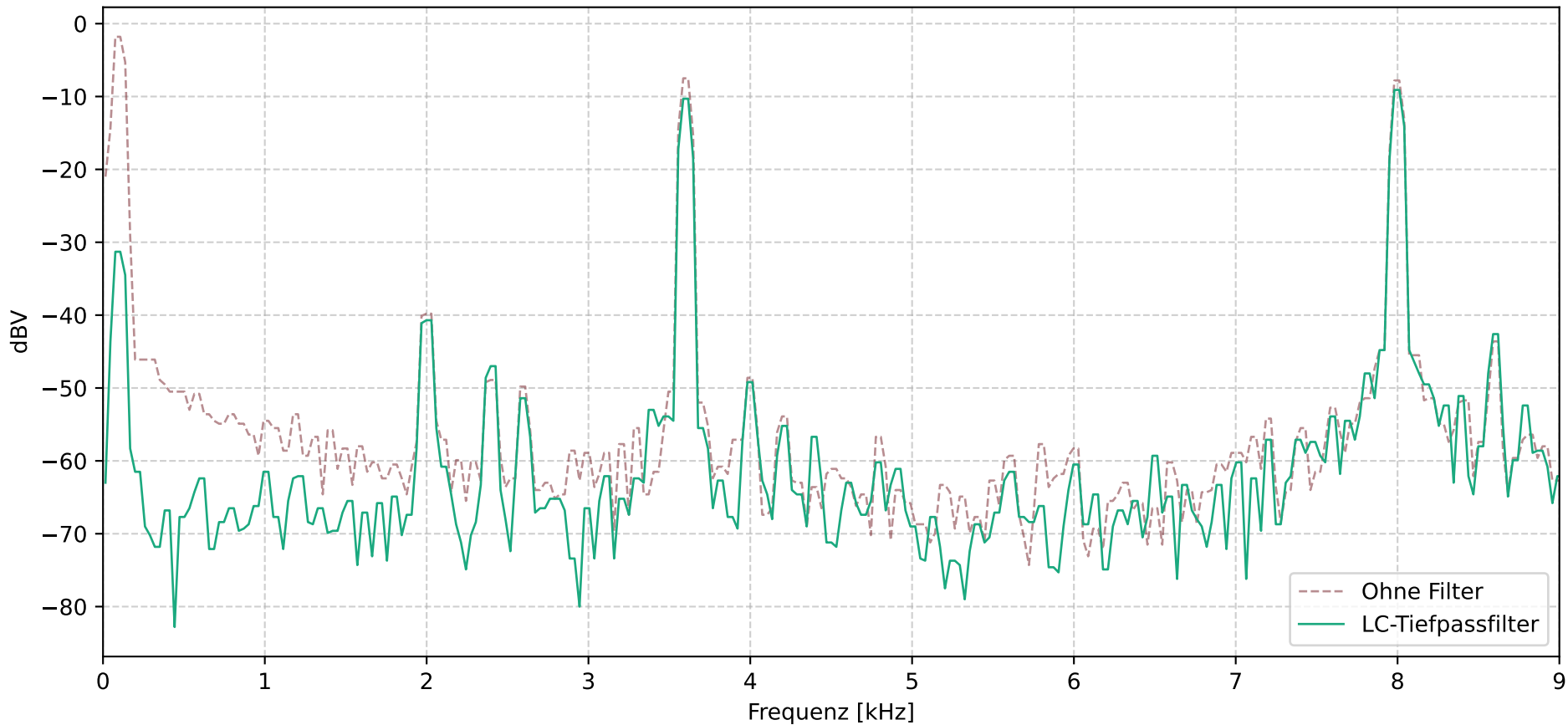
FFT Vergleich: Tiefpass vs. Ohne Filter
