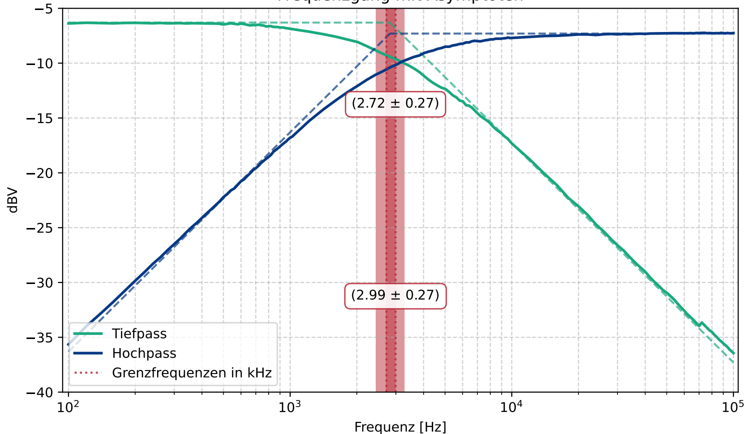
Frequenzgang mit Asymptoten
