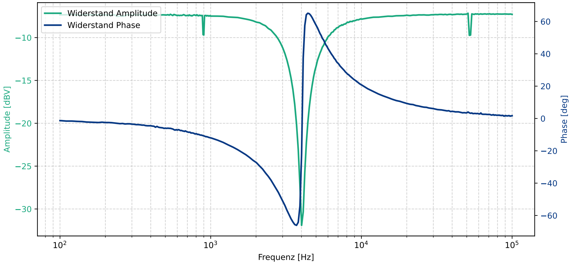
Frequenzgang und Phasengang
