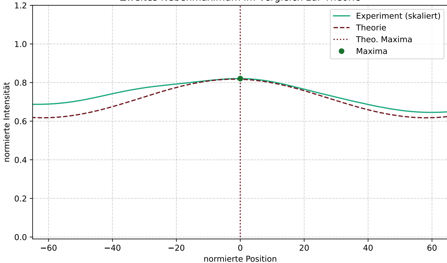
Zweites Nebenmaximum im Vergleich zur Theorie
