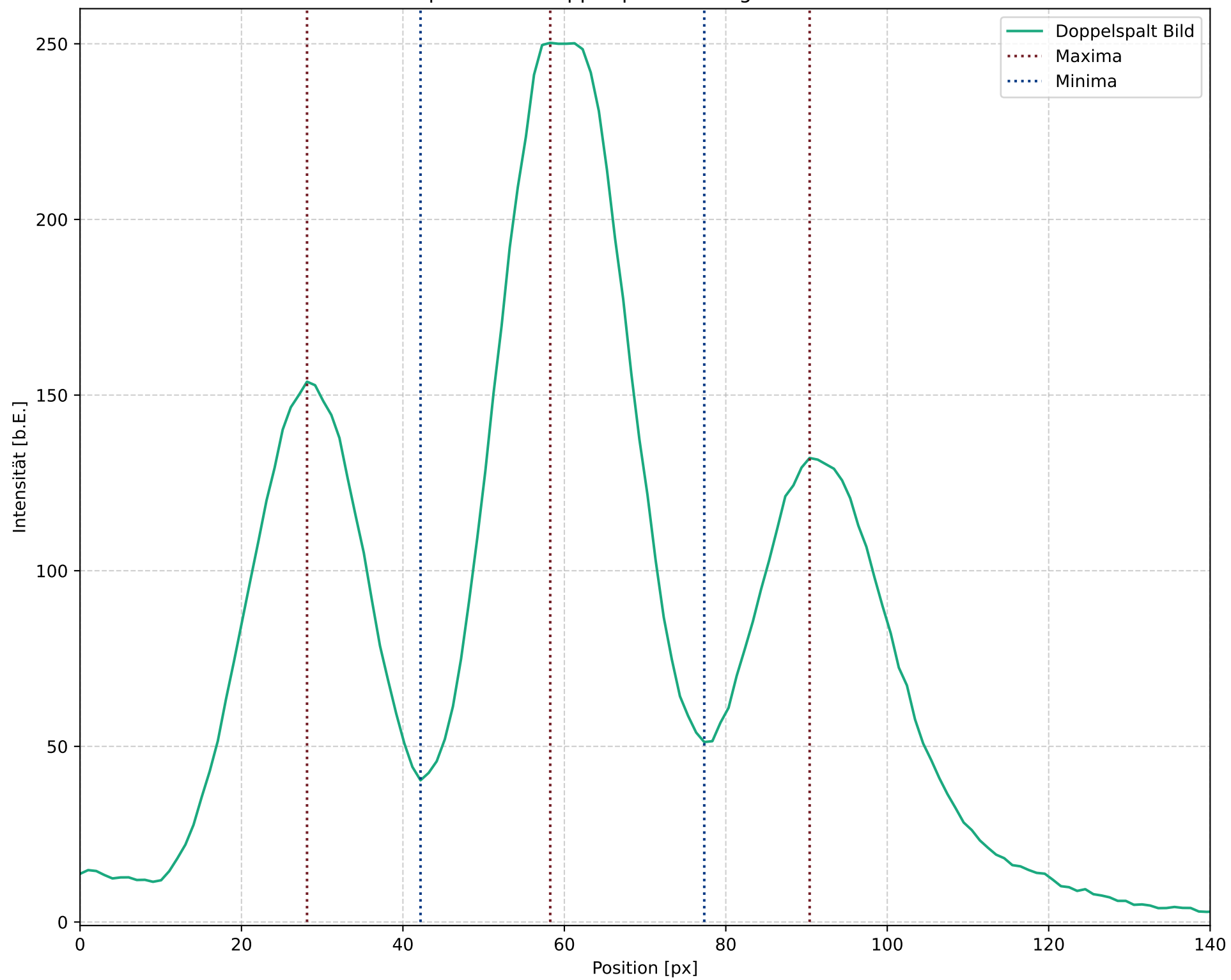
Itensitätsprofile am Doppelspalt mit eingezeichneten Extrma
