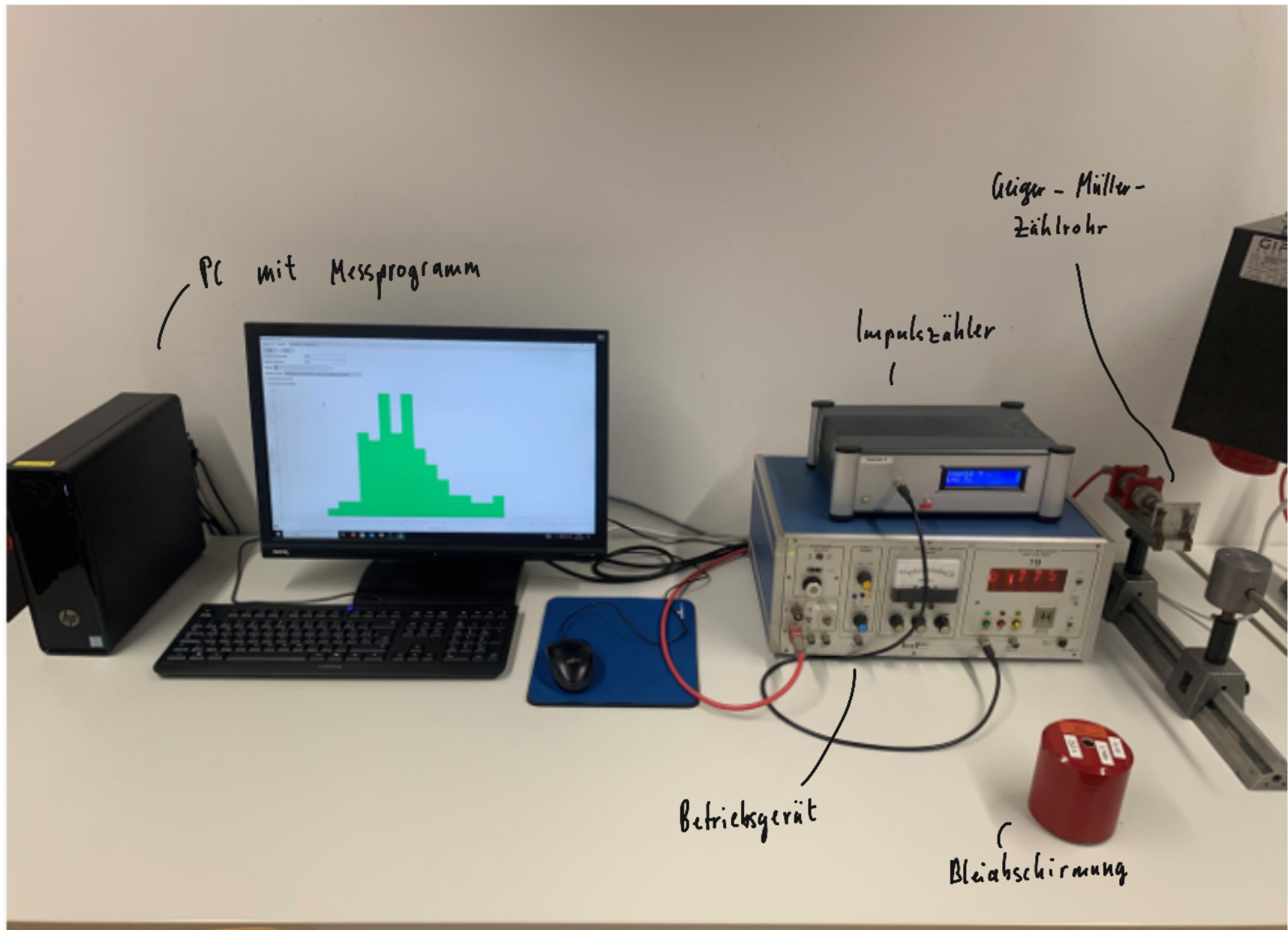
Fig. I. 1.: Beschrifteter Versuchsaufbau
