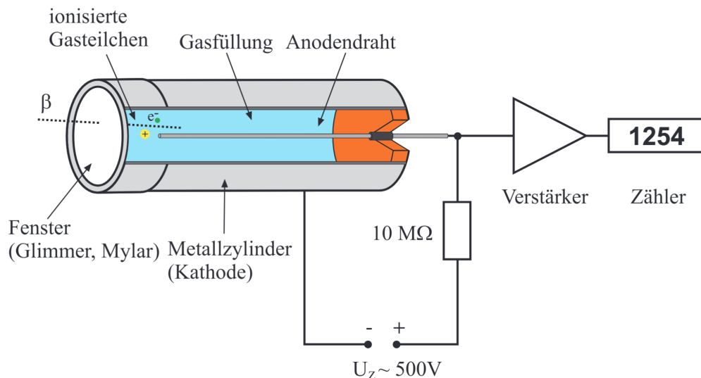
Abbildung 1.III: Schematischer Aufbau des Geiger-Müller-Zählrohrs. [Wag26b]
