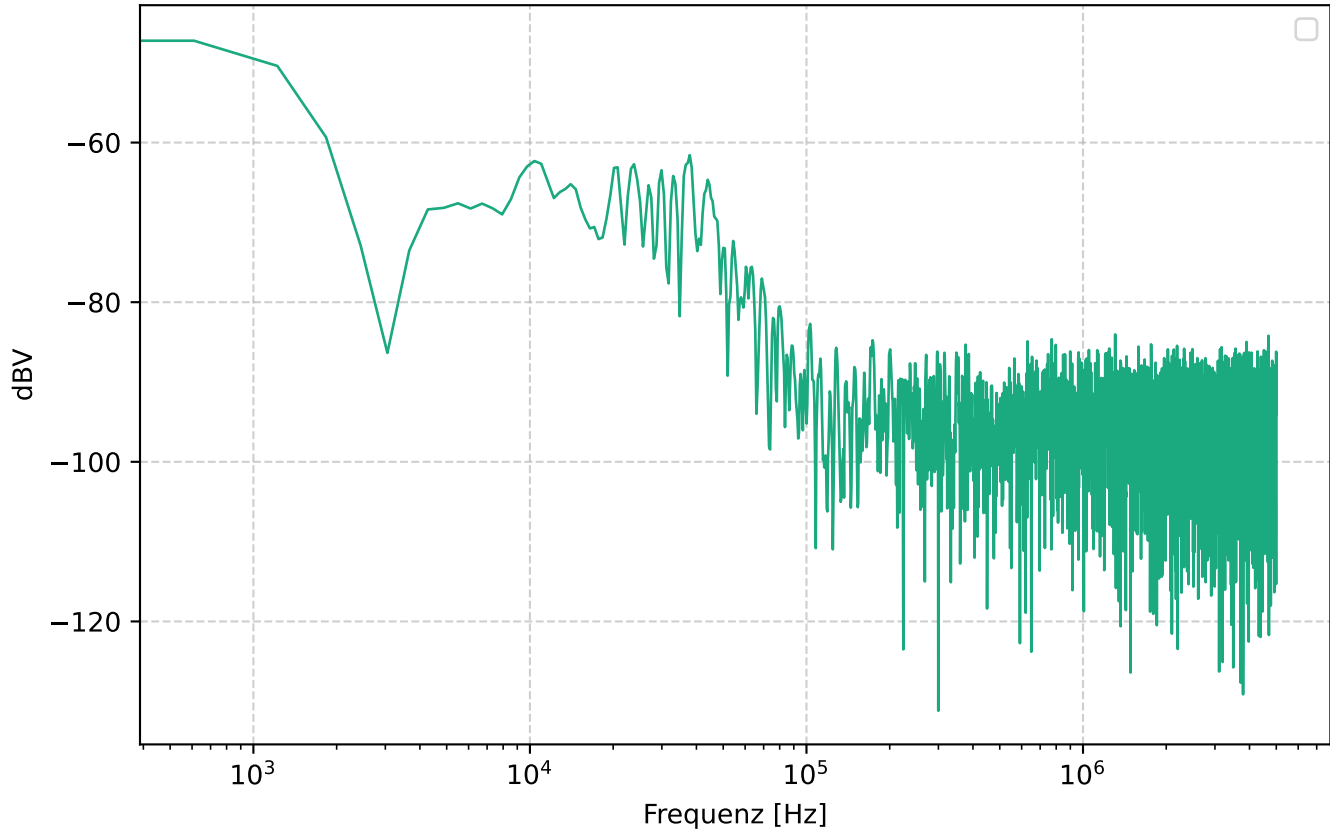
Frequenzgang mit Bandpassfilter (5k \Omega )
