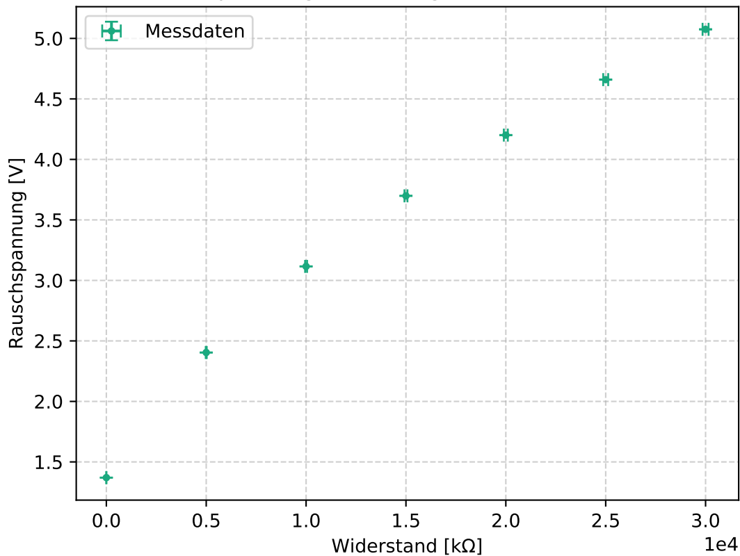
Rauschspannung in Abhängigkeit des Widerstandes
