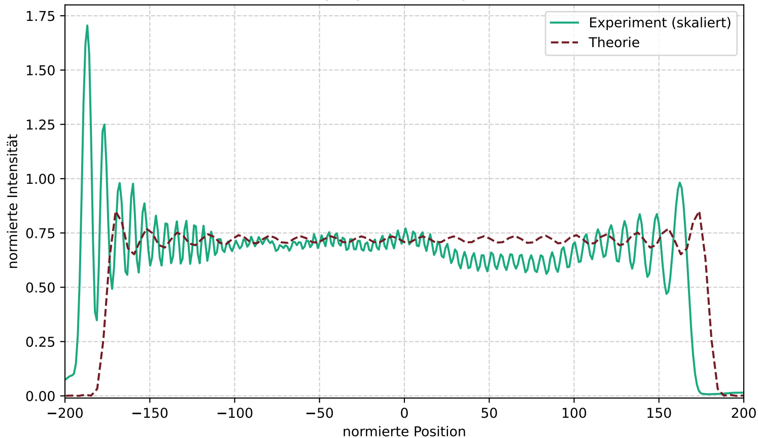
Gesamtes Beugungsbild im Vergleich zur Theorie
