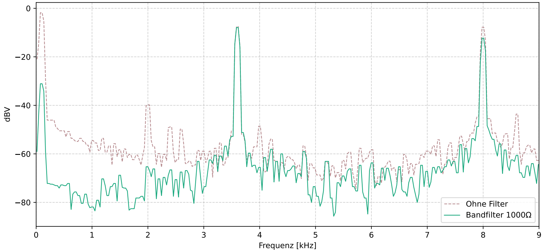
FFT Vergleich: 1000 Ohm vs. Ohne Filter
