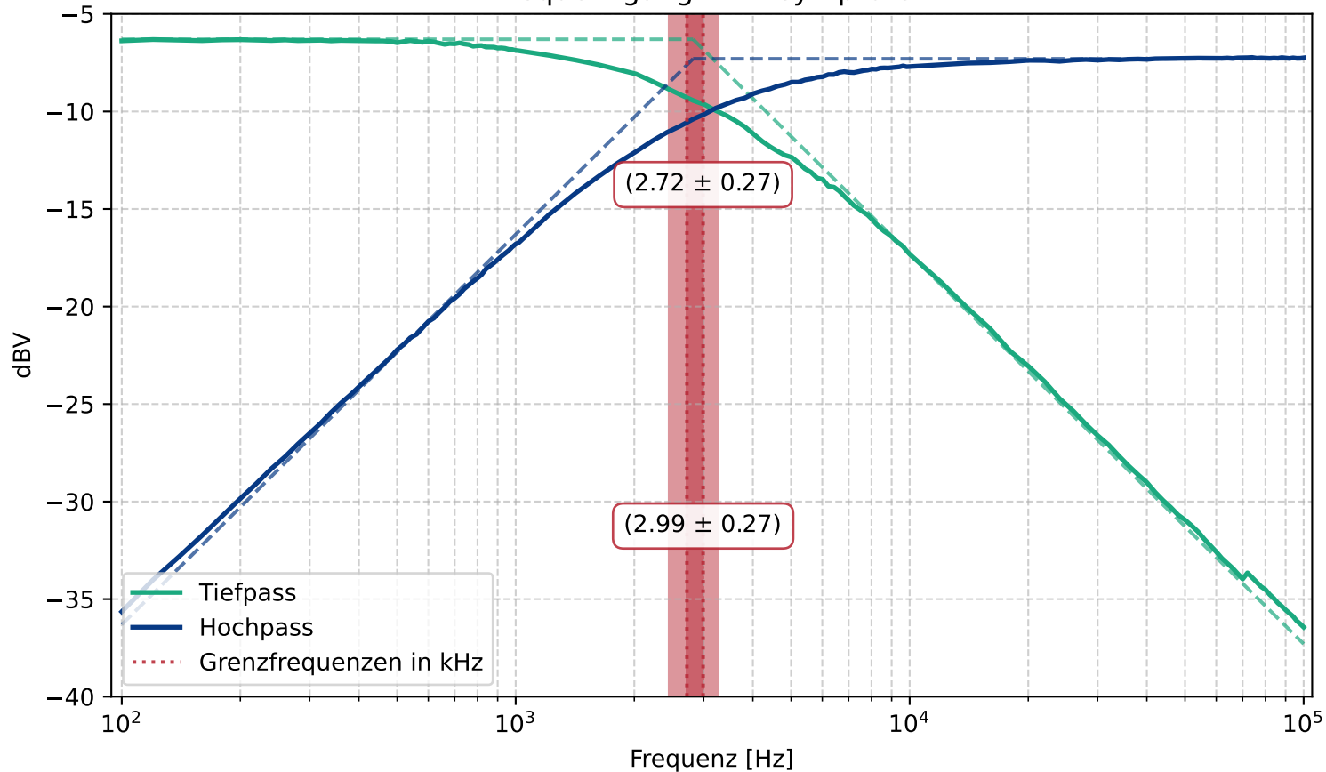
Frequenzgang mit Asymptoten
